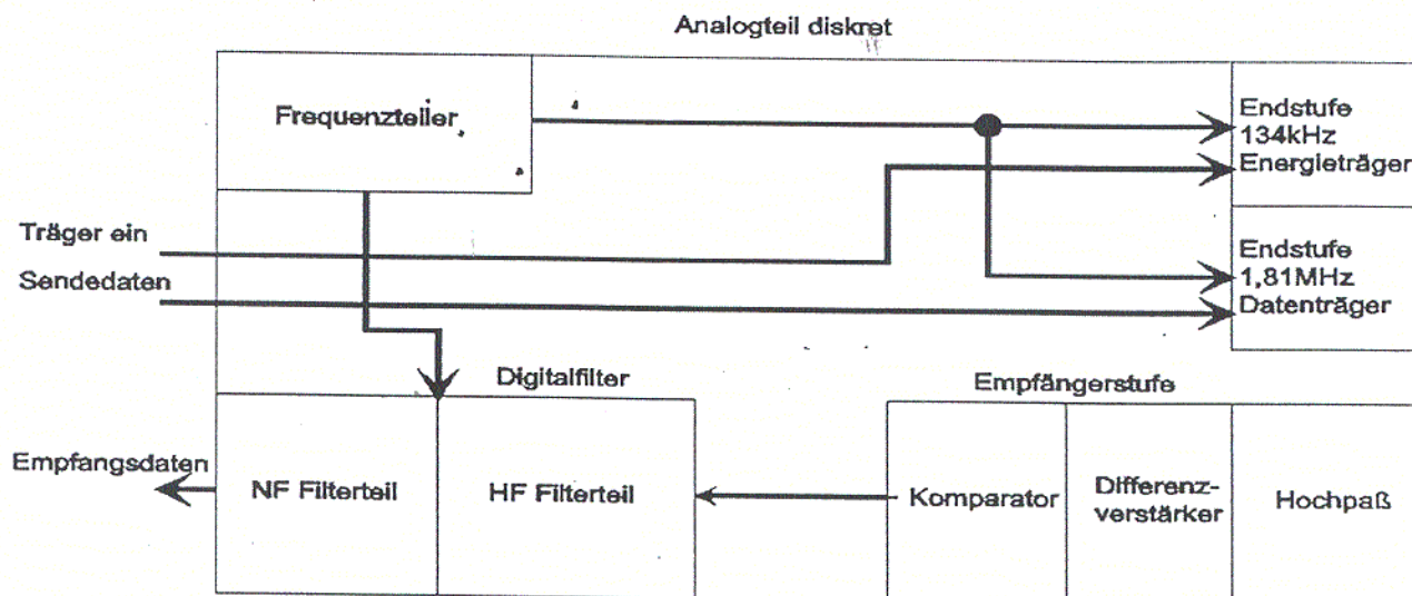
Abbildung 2 Detail Analogteil
