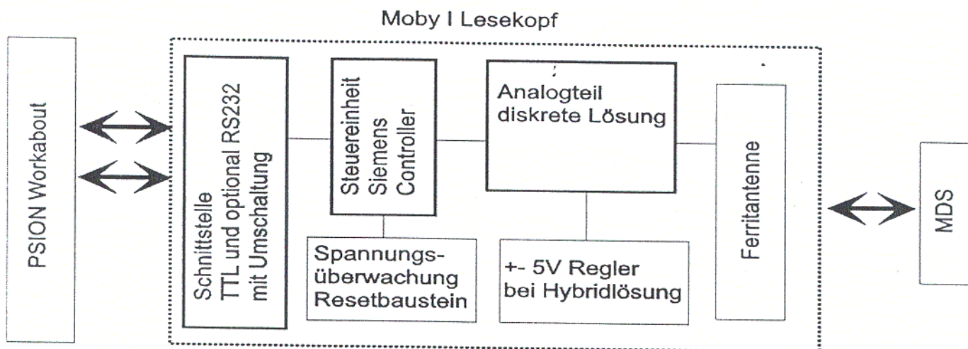
Abbildung 1 Blockschaltbild
