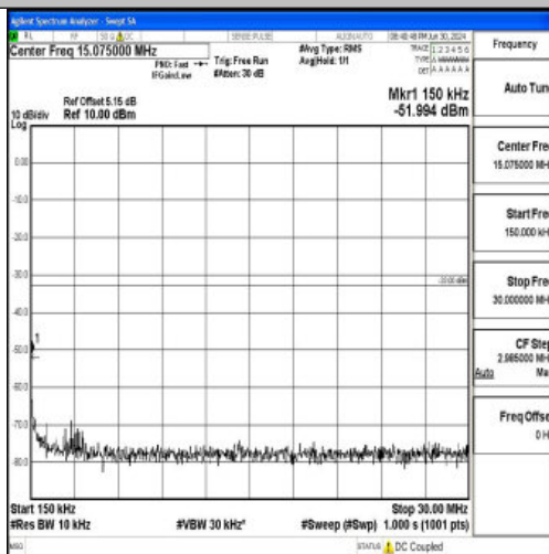
Band25 20MHz 16QAM 26140 1RB#0 0.15~30 0.15~30
