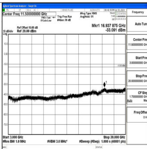
Band25 20MHz QPSK 26140 1RB#0 3000~20000 3000~20000
