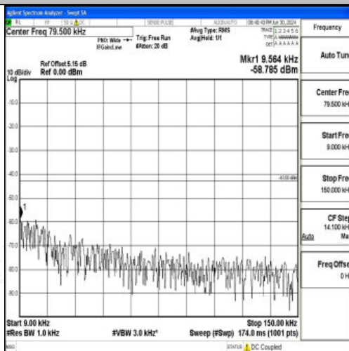
Band25 20MHz 16QAM 26140 1RB#0 0.009~0.15 0.009~0.15
