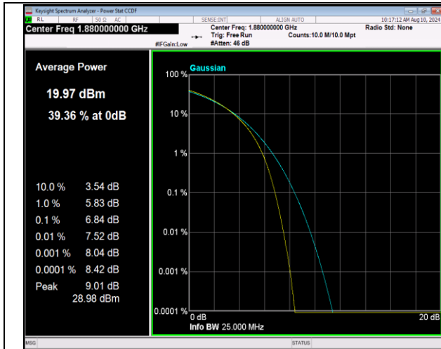
2-2-20MHz-20MHz-QPSK-QPSK-18801-18999-100RB#0-100RB#0-PASS
