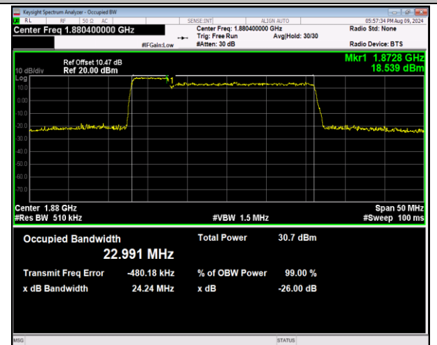
2-2-5MHz-20MHz-QPSK-QPSK-18808-18925-25RB#0-10 ORB#0-PASS
