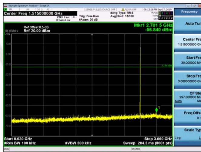
30MHz-3GHz
