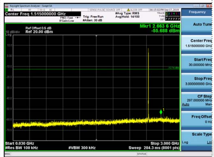
30MHz-3GHz
