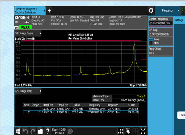
Band4-20MHz-QPSK-20300-1RB#99-PASS
