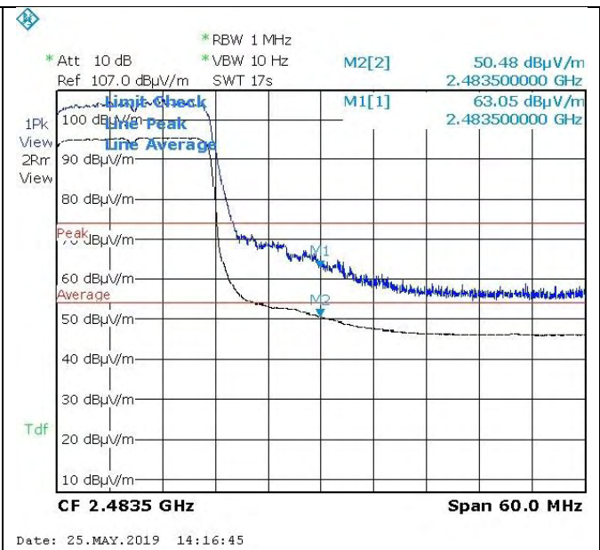
802.11n 2462M--High
