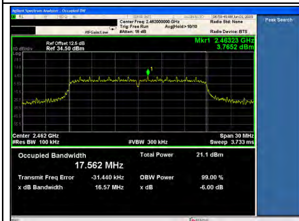
11n-20MHz-6dB BW-High-MCS0
