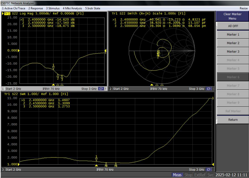
V.S.W.R
