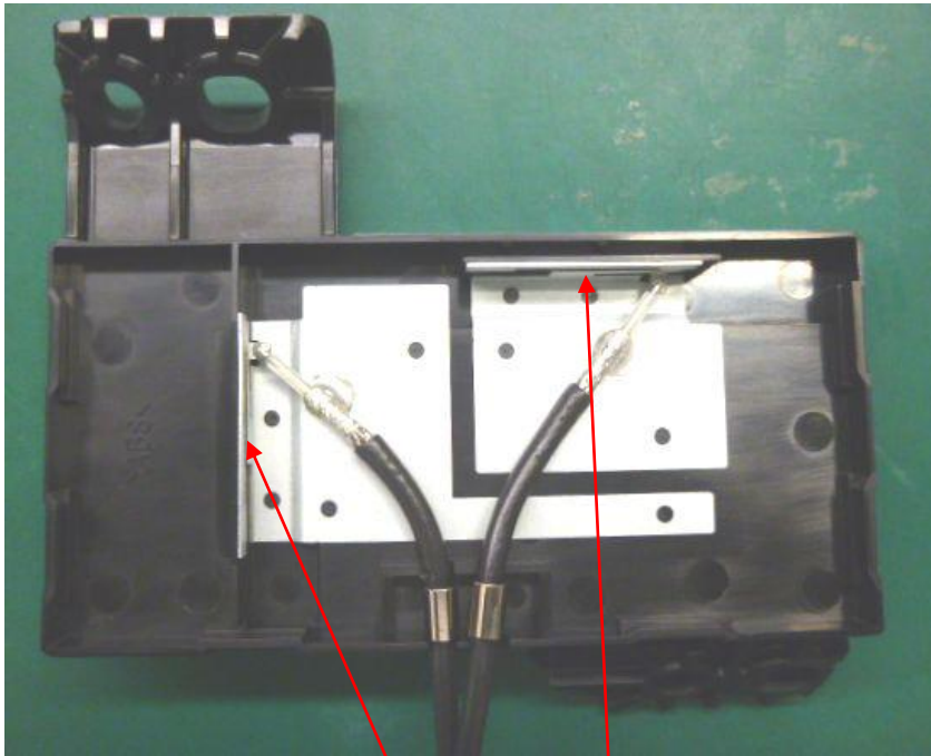
RF0 (WiFi2.4GHz, U-NII-1,U-NII-3)
