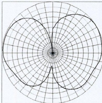
实测垂直面方向图
