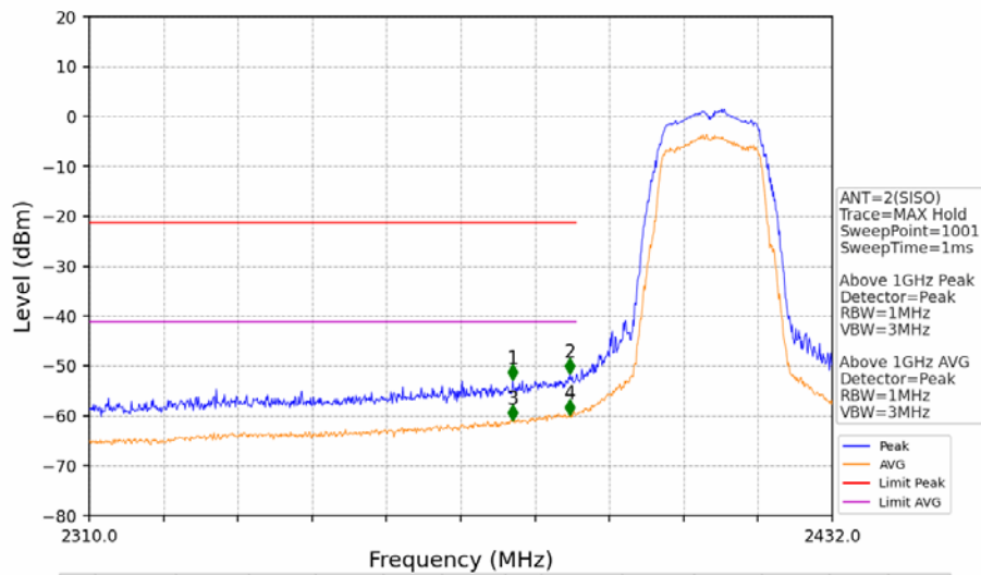
802.11g_LCH_2412MHz_Ant2 (SISO)_NTNV
