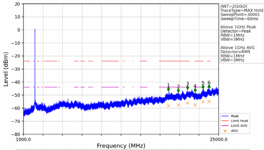
802.11g_LCH_2412MHz_Ant2 (SISO)_NTNV
