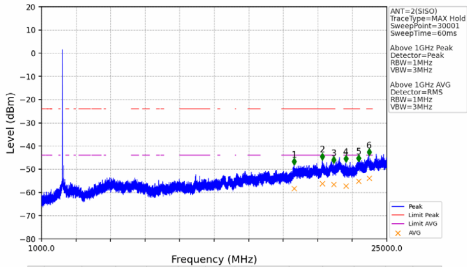
802.11b_HCH_2462MHz_Ant2 (SISO)_NTNV
