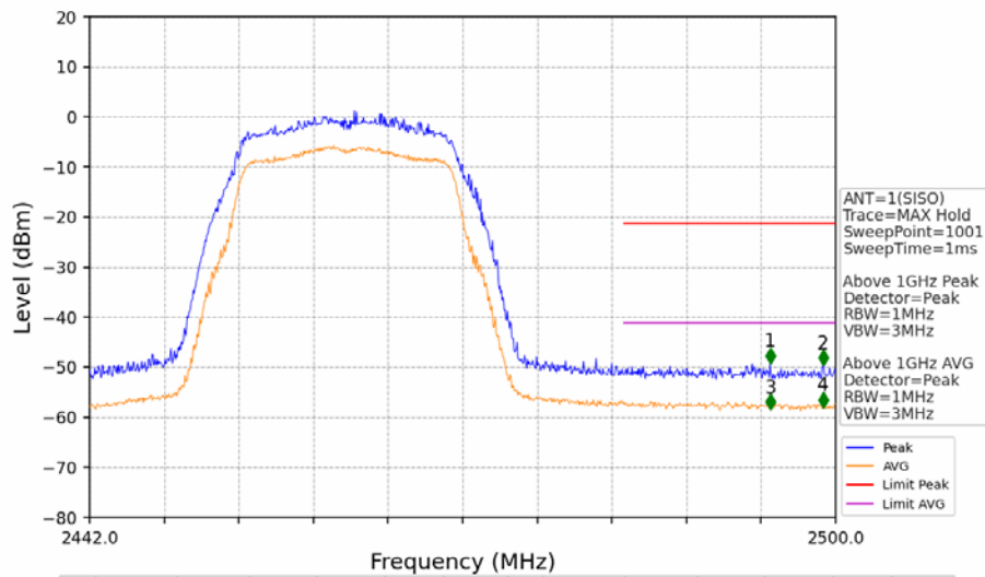
802.11g_HCH_2462MHz_Ant1 (SISO)_NTNV
