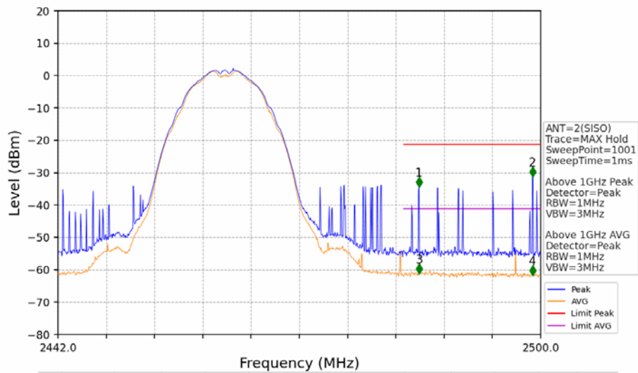
802.11b_HCH_2462MHz_Ant2 (SISO)_NTNV
