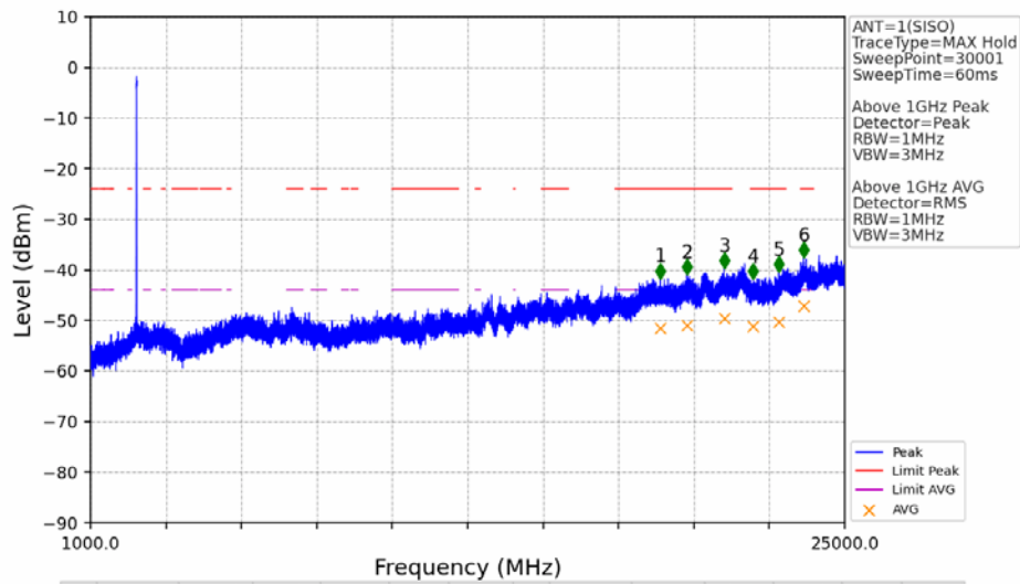
802.11g_HCH_2462MHz_Ant1 (SISO)_NTNV
