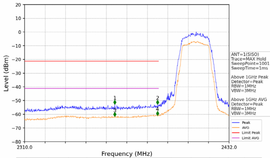
802.11g_LCH_2412MHz_Ant1 (SISO)_NTNV
