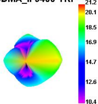
WCDMA_II 9400 TRP
