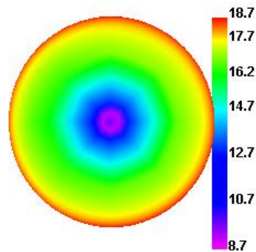
LTE71 133422 TRP
