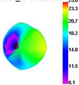
WCDMA_IV 1312 TRP
