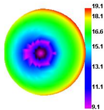
LTE12 23130 TRP
