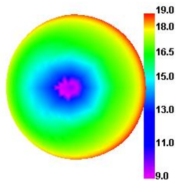
LTE12 23060 TRP
