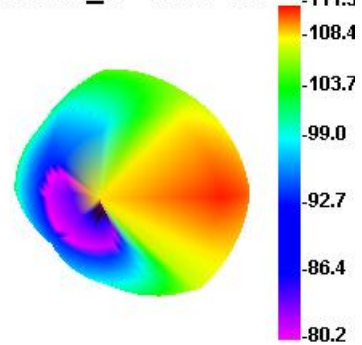
WCDMA_IV 1738 TIS
