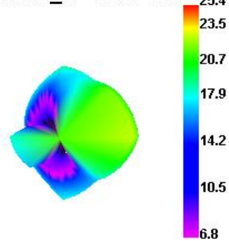
WCDMA_IV 1513 TRP
