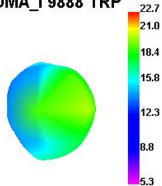
WCDMA_I 9888 TRP
