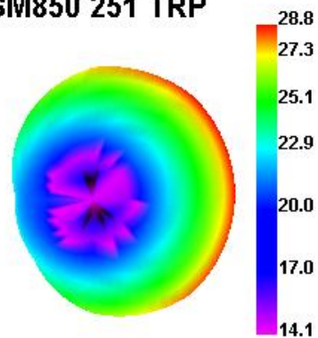
GSM850 251 TRP
