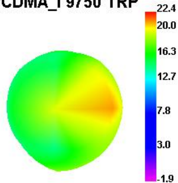
WCDMA_I 9750 TRP
