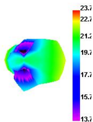
LTE2 19150 TRP
