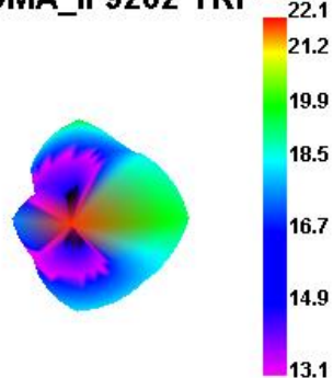
WCDMA_II 9262 TRP
