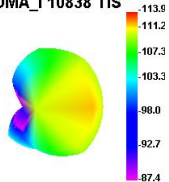
WCDMA_I 10838 TIS
