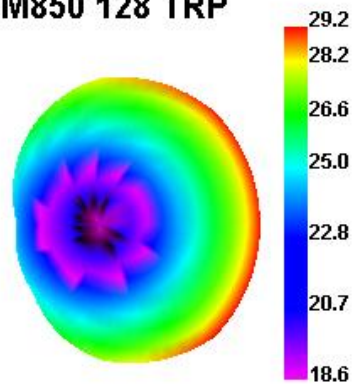
GSM850 128 TRP
