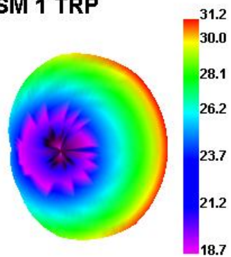
EGSM 1 TRP
