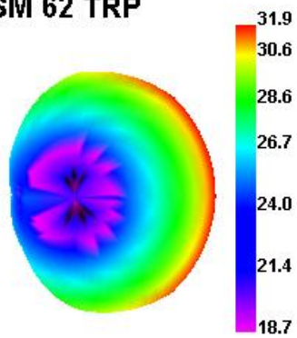
EGSM 62 TRP
