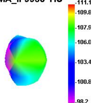
WCDMA_II 9938 TIS
