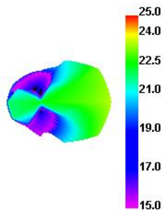
LTE2 18650 TRP
