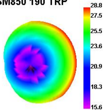
GSM850 190 TRP
