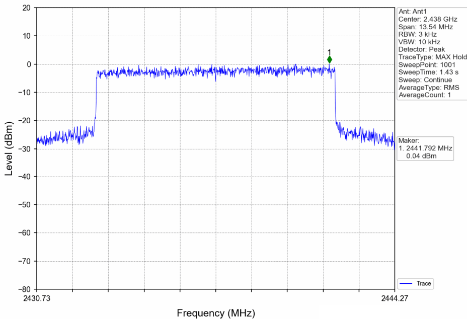
10MHz BW_MCH_2437.5MHz_Ant1_NTNV
