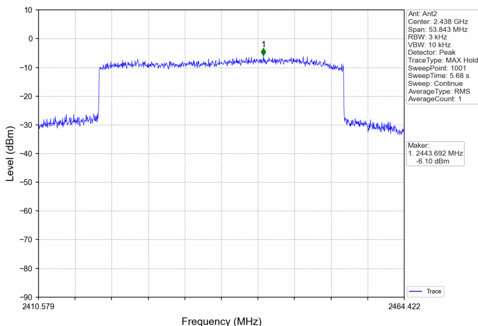
40MHz BW_MCH_2437.5MHz_MIMO_NTNV
