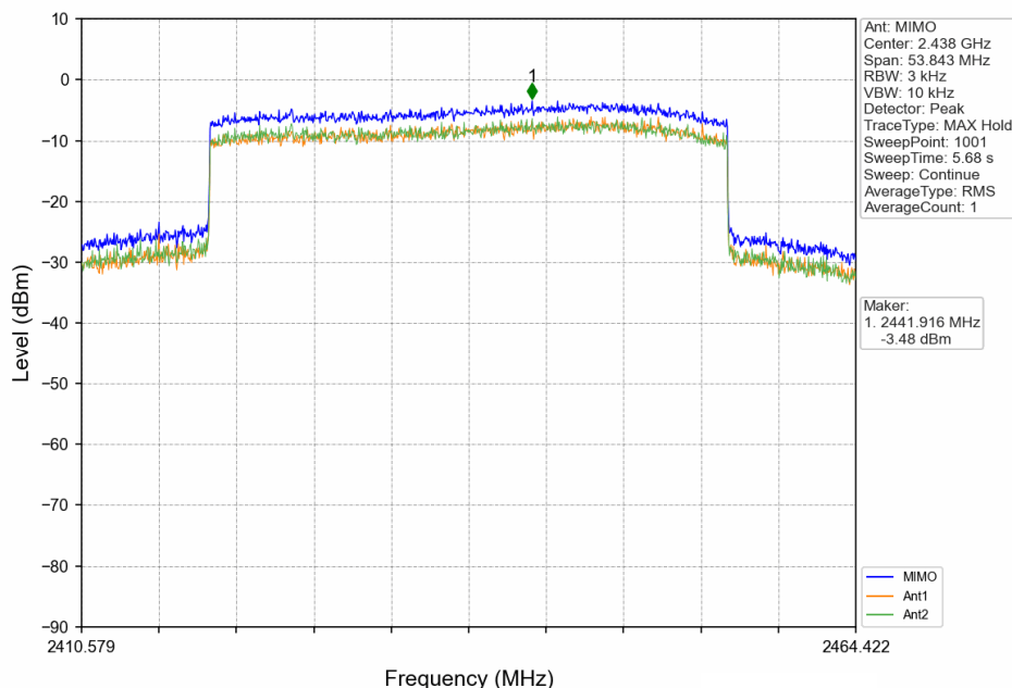
40MHz BW_MCH_2437.5MHz_MIMO_NTNV
