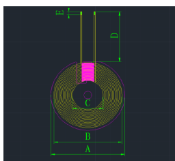
一、尺寸 DIMENSION:(mm)
