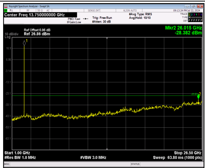
Band41-5MHz-QPSK-41215-1RB#0-Range2:1000~265 00MHz
