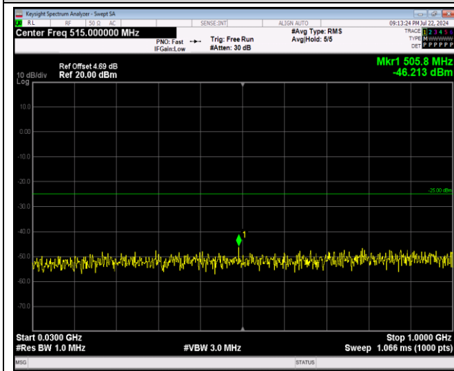
Band41-5MHz-QPSK-41215-1RB#0-Range1:30~100 OMHz
