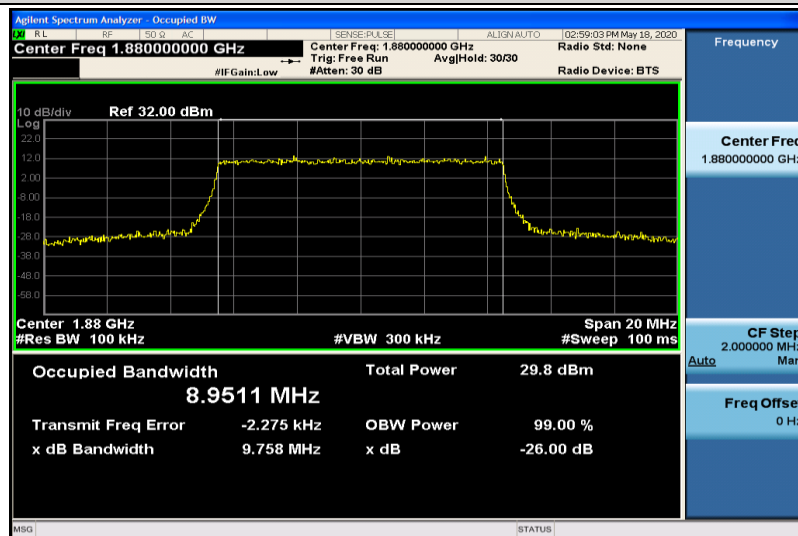
Band2-10MHz-QPSK-18900-50RB#0-8.9511
