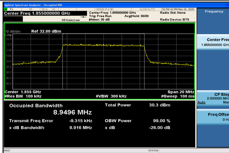
Band2-10MHz-QPSK-18650-50RB#0-8.9496
