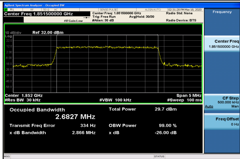
Band2-3MHz-QPSK-18615-15RB#0-2.6827
