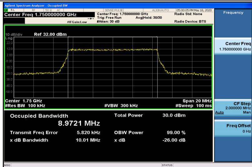
Band4-10MHz-QPSK-20350-50RB#0-8.9721
