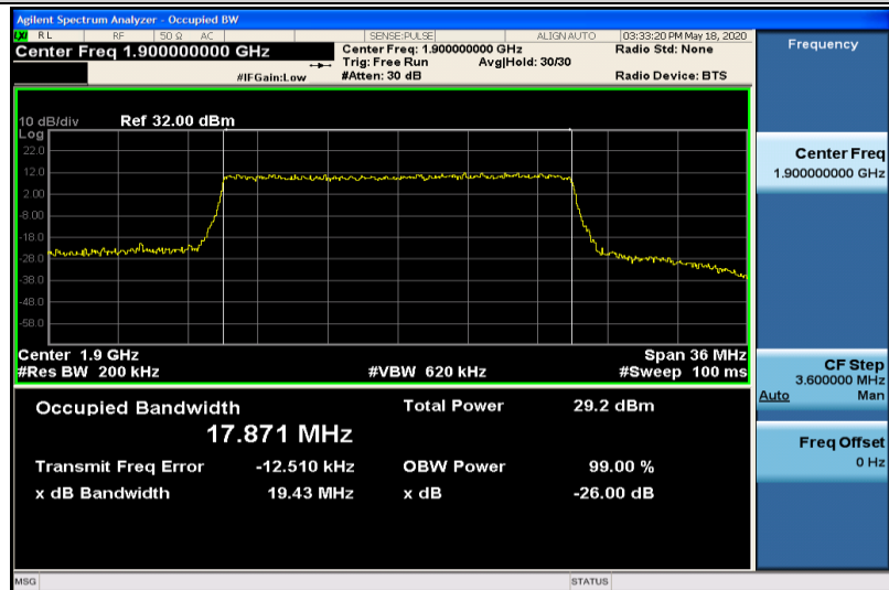
Band2-20MHz-16QAM-19100-100RB#0-17.871
