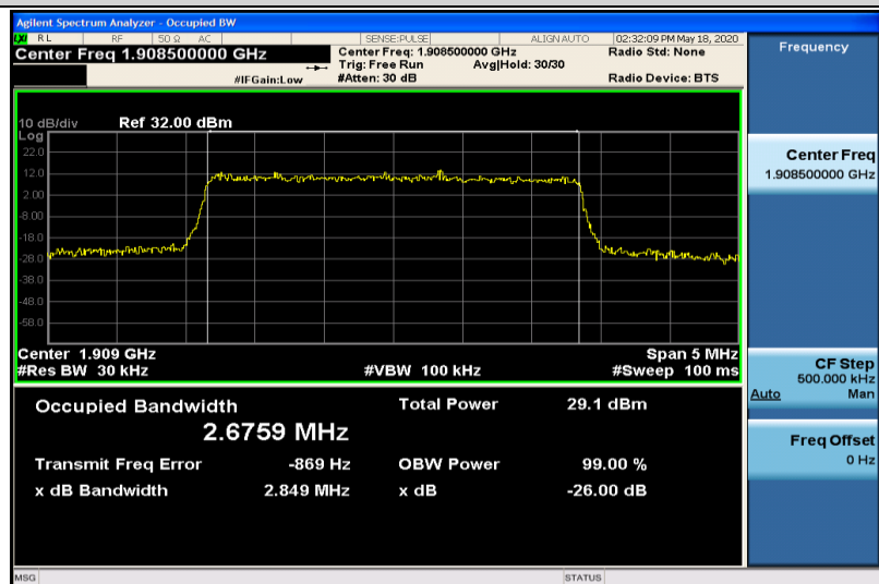
Band2-3MHz-QPSK-19185-15RB#0-2.6759
