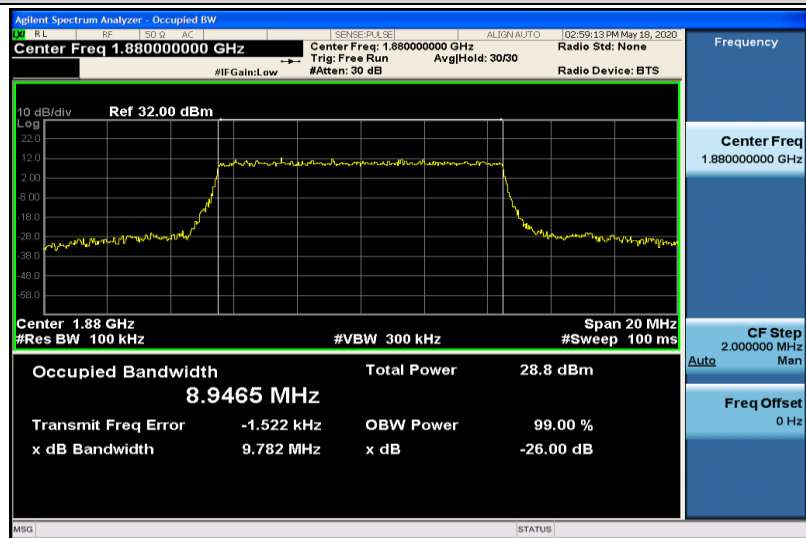
Band2-10MHz-16QAM-18900-50RB#0-8.9465
