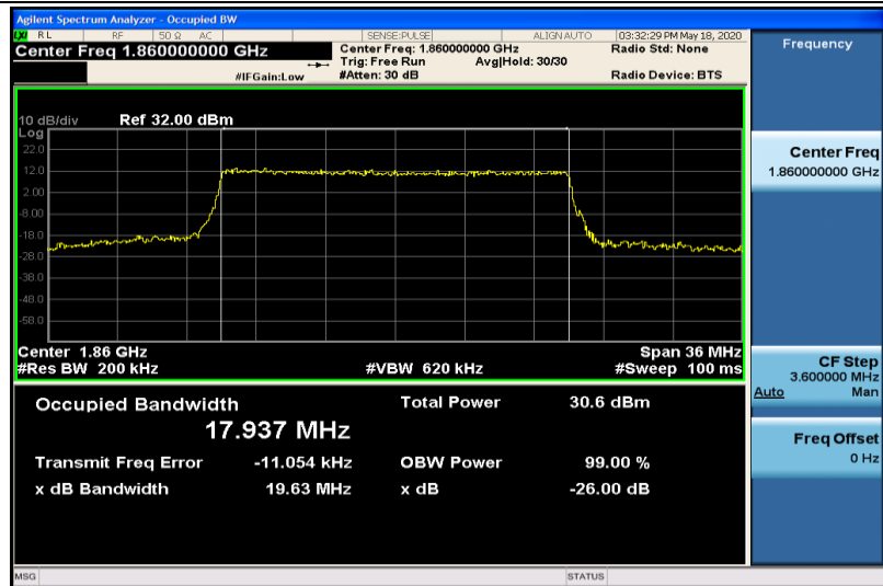
Band2-20MHz-QPSK-18700-100RB#0-17.937
