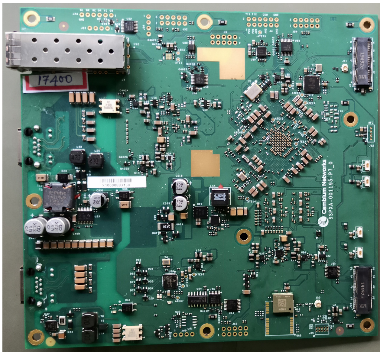
V3000 SSAXA-001000 PCBA Bottom View
