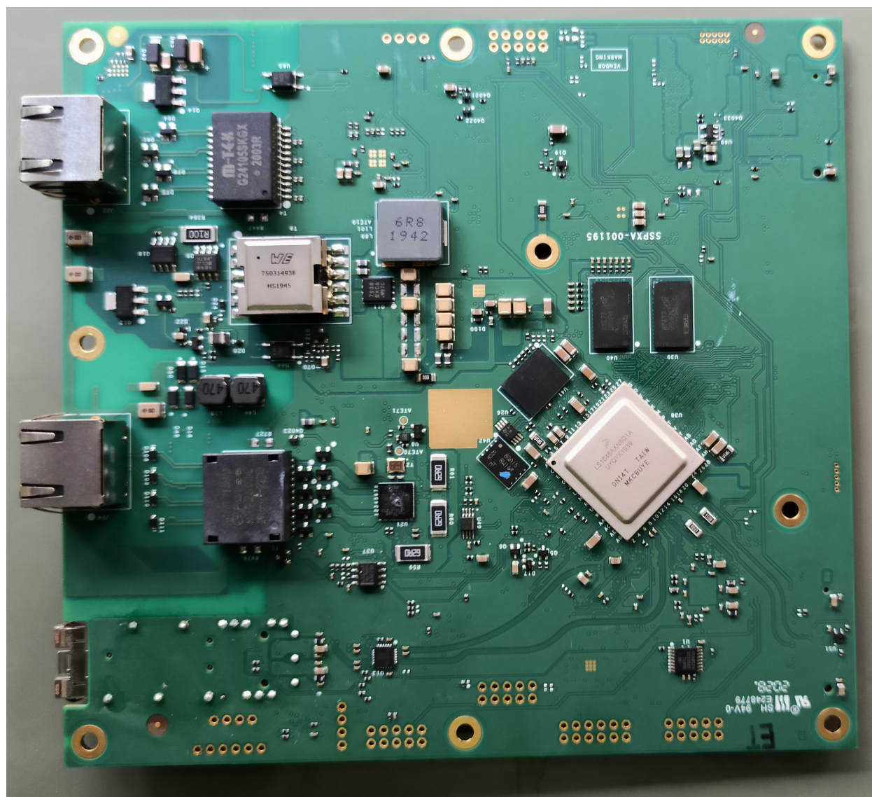
V3000 SSAXA-001000 PCBA Top View
