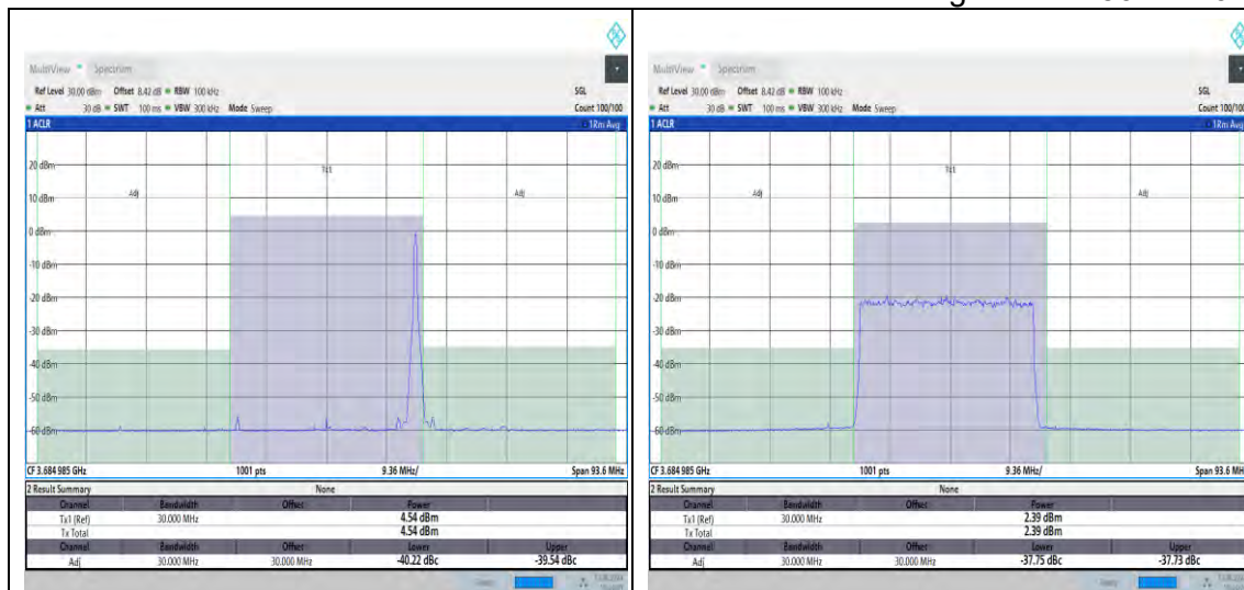
NTNV_N48_PC3_30_30_H_TID12_#1_-30_30
