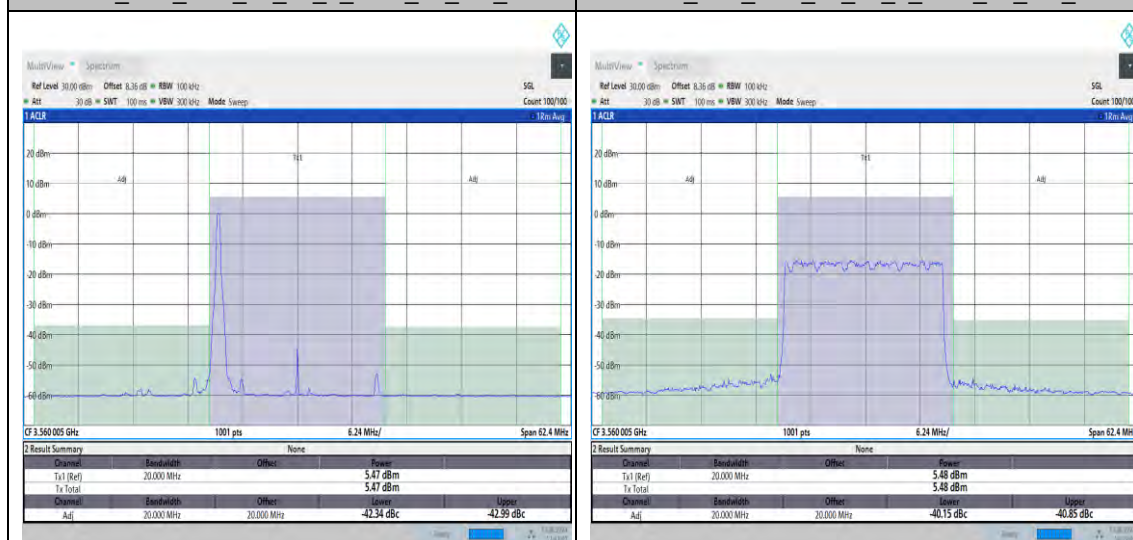
NTNV_N48_PC3_30_20_L_TID2_#1_+20_20
