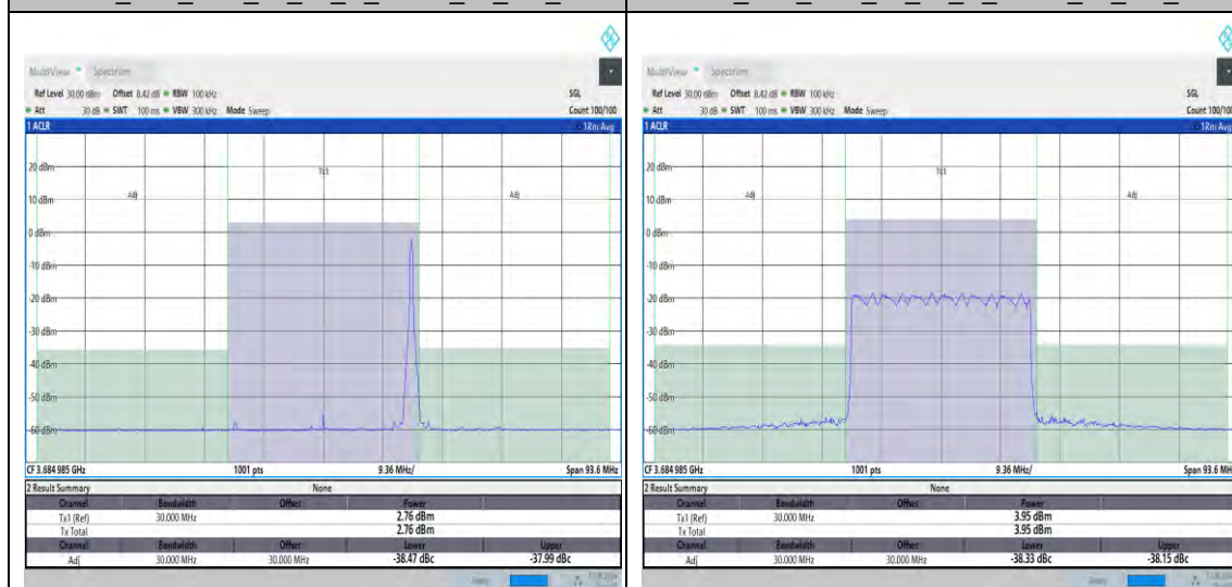
NTNV_N48_PC3_30_30_H_TID15_#1_-30_30
