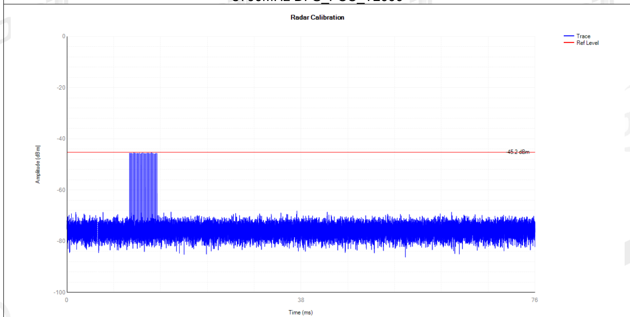
5700MHz DFS_FCC_T3000
