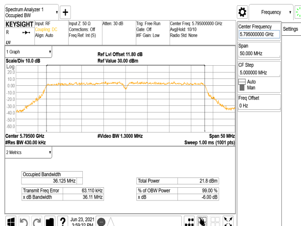
802.11n_40MHz_Test_Chain0
