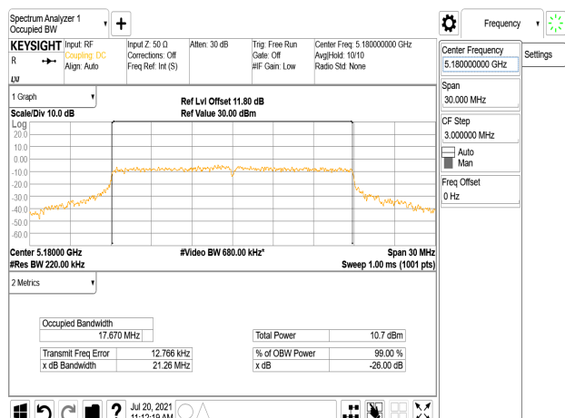
802.11n_20MHz_Chain1_5180MHz
