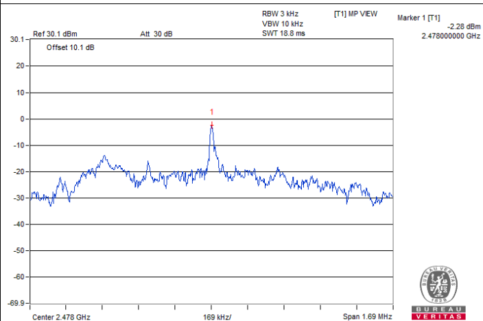
logi bolt-2M : CH 38
