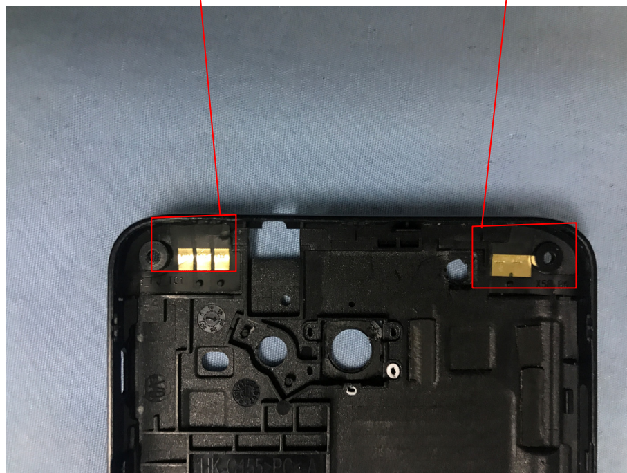
LTE_Rx Ant.
