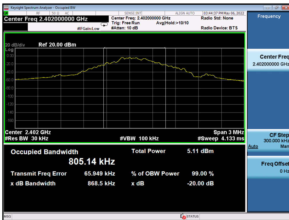
GFSK 2402MHz
