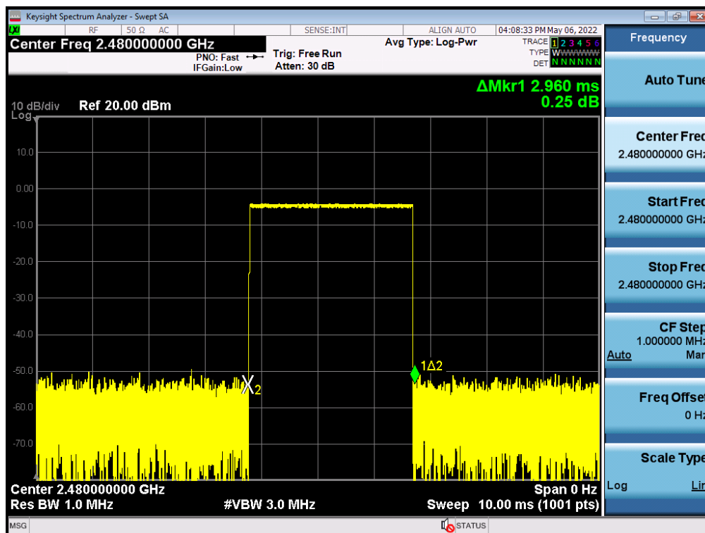
GFSK 2480MHz
