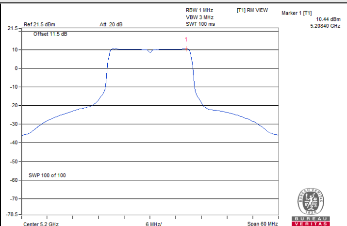
802.11be (EHT20) / Chain 3 : CH 40
