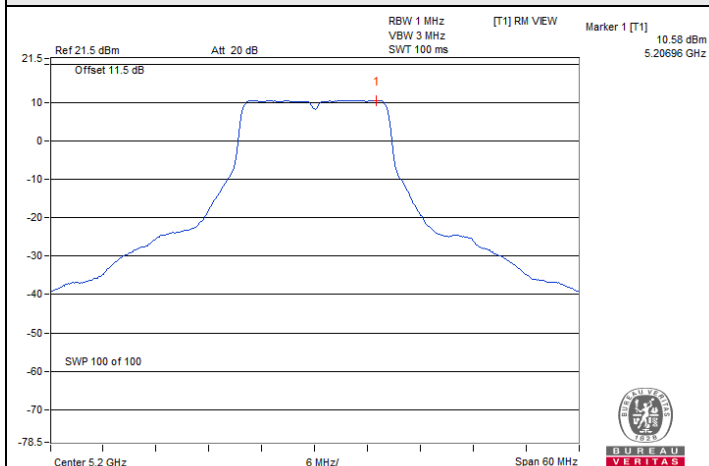
802.11a / Chain 3 : CH 40
