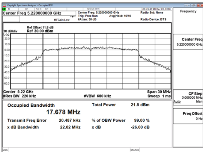
802.11n_20MHz_Chain1_5220MHz
