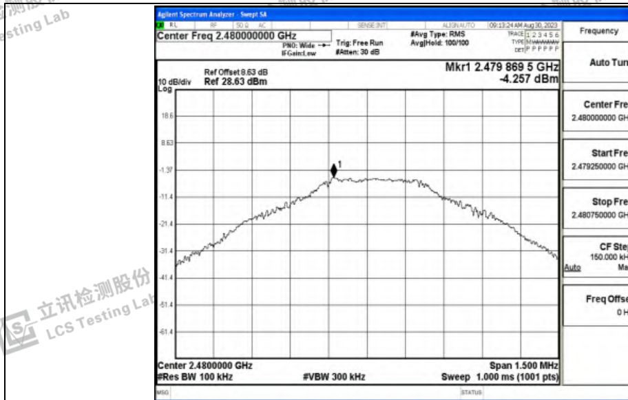
DH5_Ant_2480_30~1000
