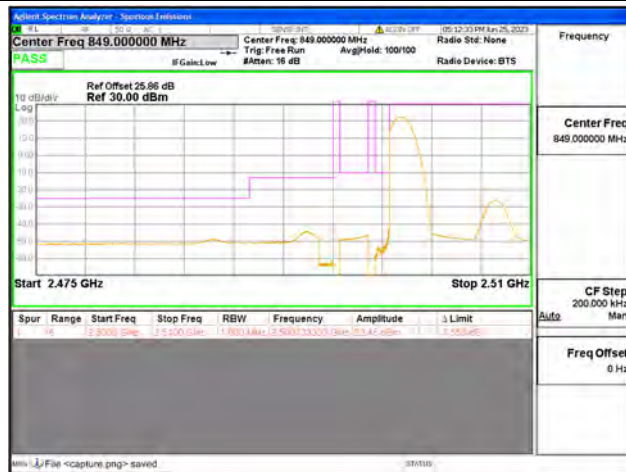
Band7 / 15MHz / Low CH / QPSK / 1 RB
