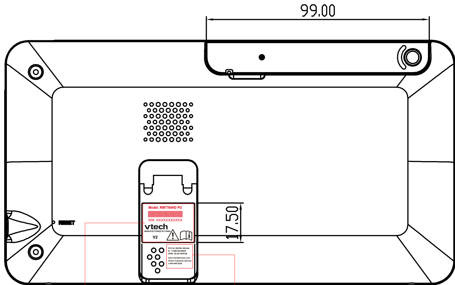
Label 22.6x17mm
