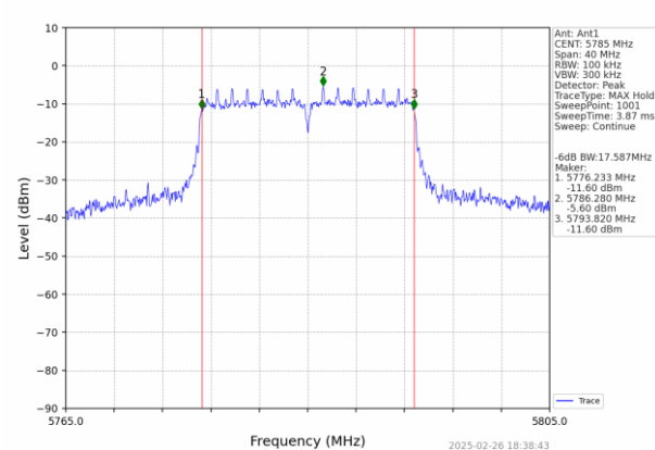
802.11n(HT20)_MCH_5785MHz_Ant1_NTNV
