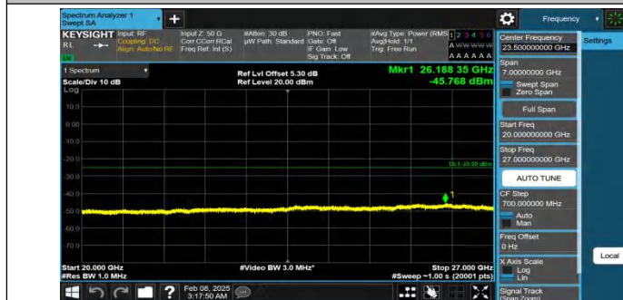
Band38-20MHz-QPSK-37850-1RB#0-20000~27000-PASS
