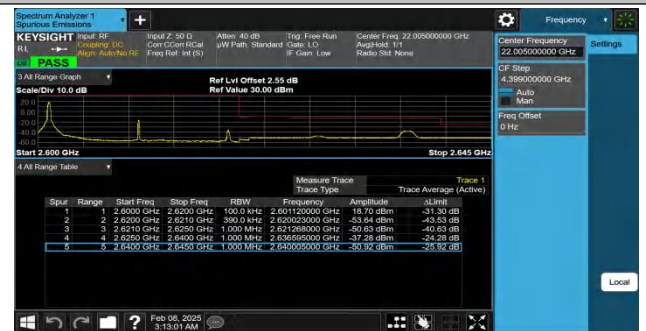
Band38-20MHz-QPSK-38150-1RB#0-PASS
