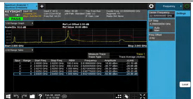
Band38-20MHz-QPSK-38150-1RB#99-PASS
