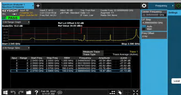
Band38-20MHz-QPSK-37850-1RB#99-PASS
