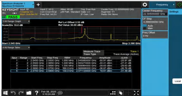
Band38-20MHz-QPSK-37850-1RB#0-PASS
