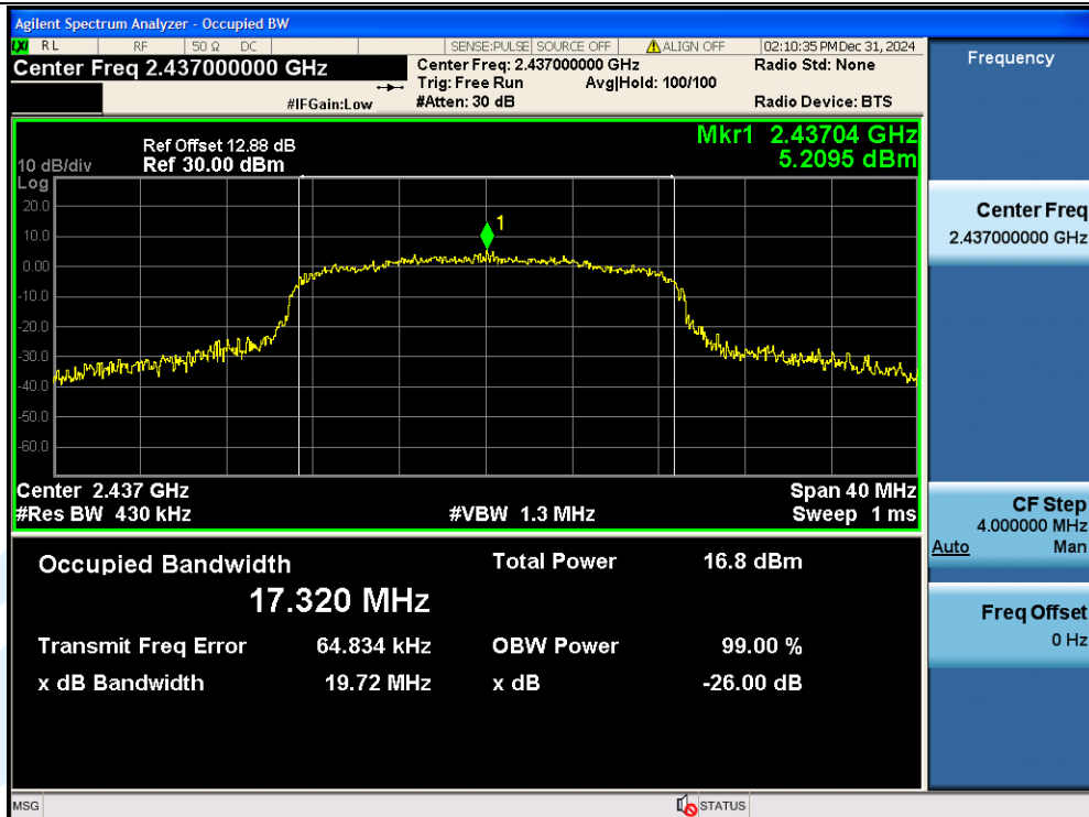
11G-Ant1-2437
