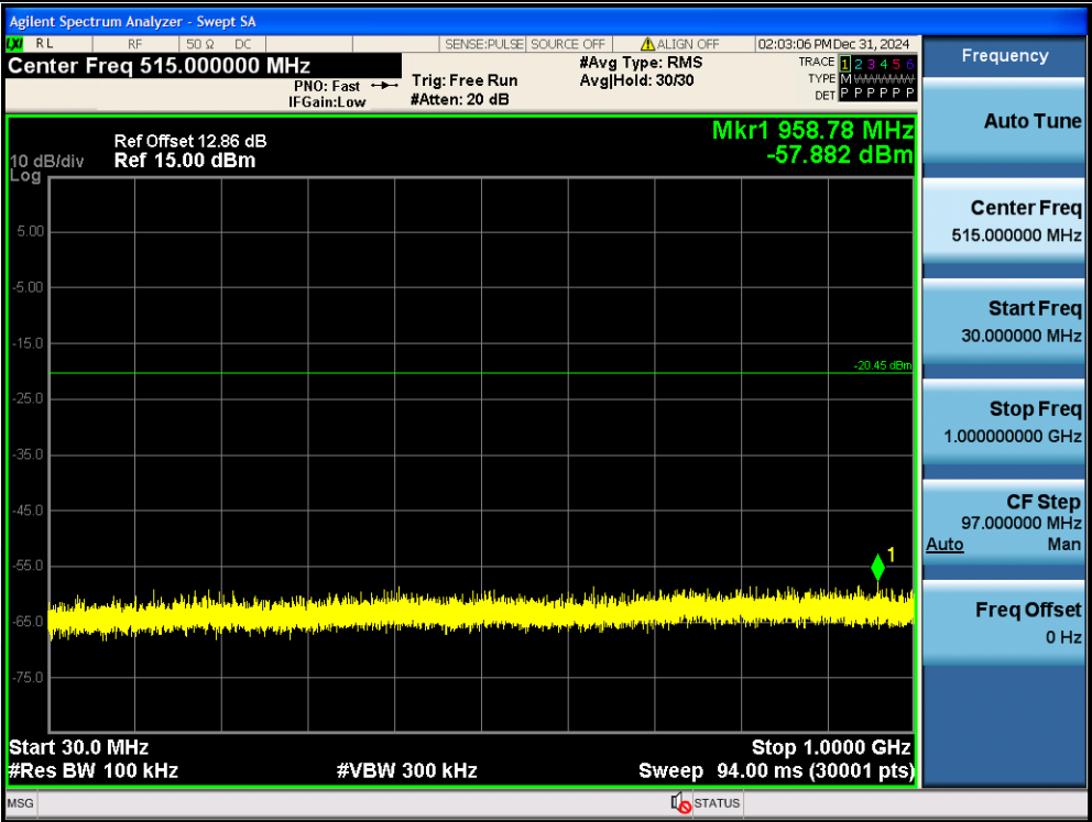
11G-Ant1-2412-30~1000-PASS
