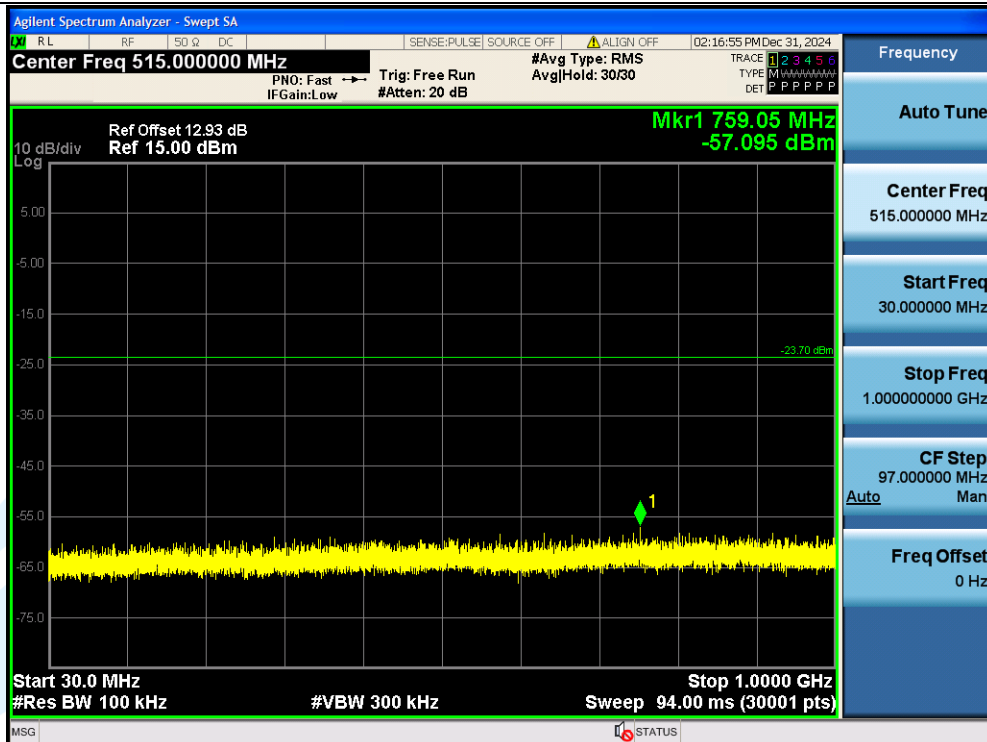
11G-Ant1-2462-30~1000-PASS
