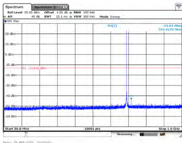
15 kHz / BPSK / CH134082 / 1RB0 / Below 1 GHz
