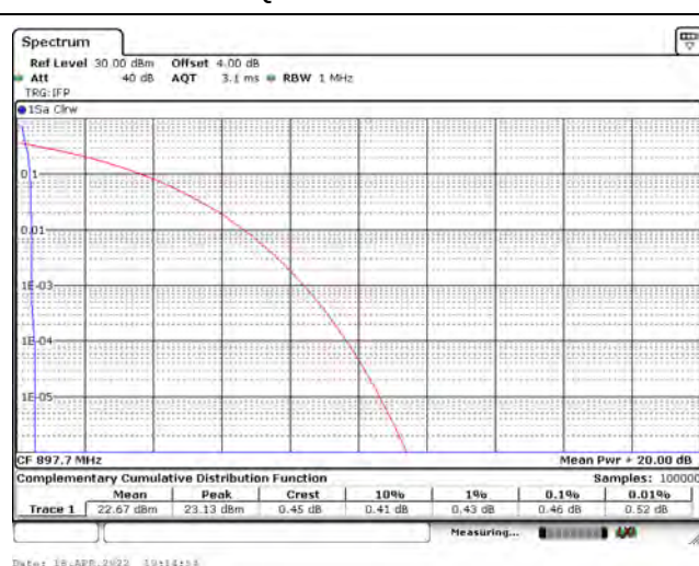
15 kHz / QPSK / CH21627 / 1RB0
