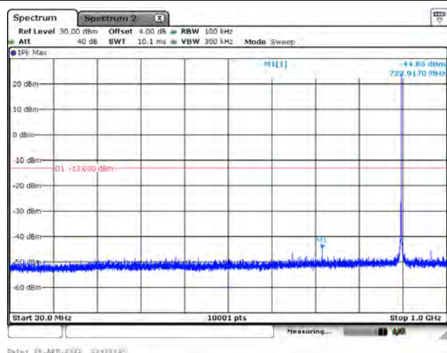
3.75 kHz / QPSK / CH21653 / 1RB47 / Below 1 GHz
