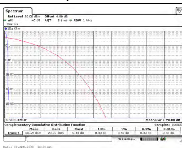
15 kHz / QPSK / CH21653 / 1RB11
