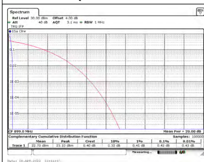
15 kHz / QPSK / CH21640 / 1RB0
