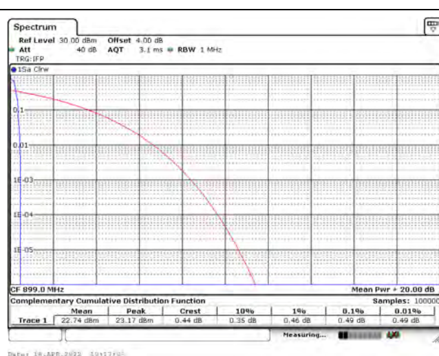
15 kHz / BPSK / CH21640 / 1RB0
