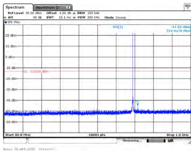
3.75 kHz / QPSK / CH134082 / 1RB0 / Below 1 GHz
