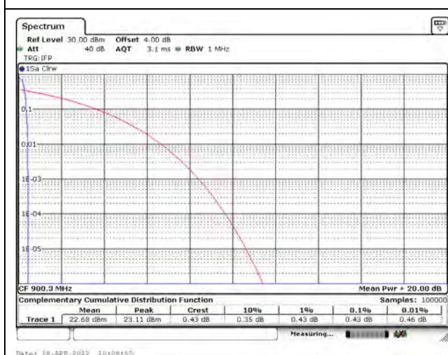
15 kHz / BPSK / CH21653 / 1RB11
