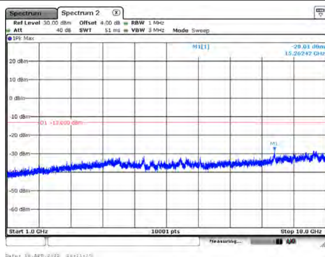
15 kHz / BPSK / CH134180 / 1RB11 / Above 1 GHz
