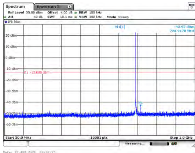
15 kHz / QPSK / CH134082 / 1RB0 / Below 1 GHz
