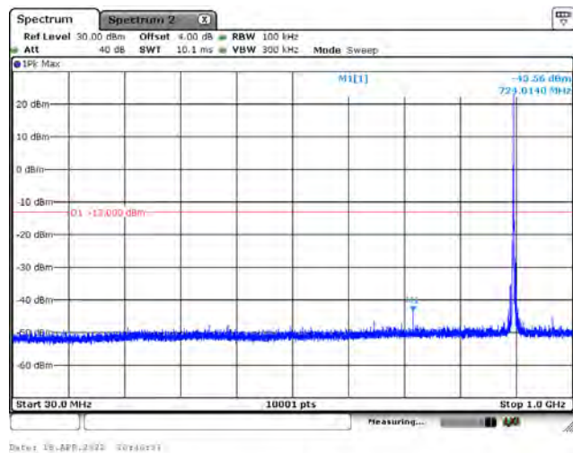
15 kHz / BPSK / CH21640 / 1RB0 / Below 1 GHz
