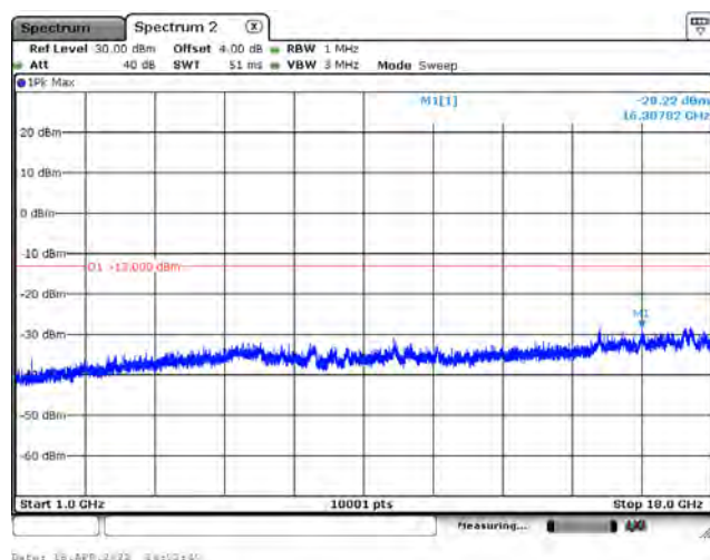
15 kHz / BPSK / CH134082 / 1RB0 / Above 1 GHz
