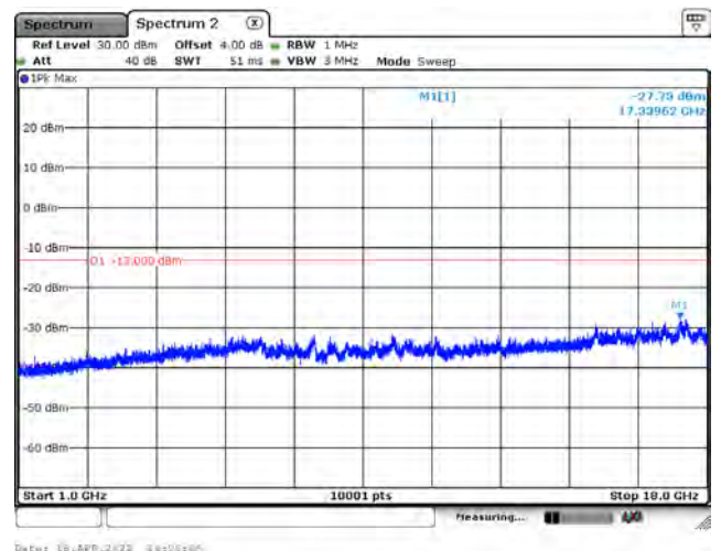
15 kHz / QPSK / CH134082 / 1RB0 / Above 1 GHz
