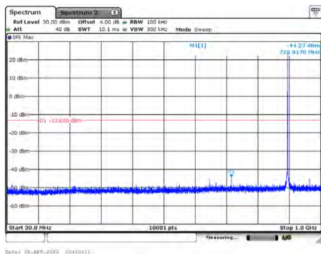
3.75 kHz / QPSK / CH21640 / 1RB0 / Below 1 GHz
