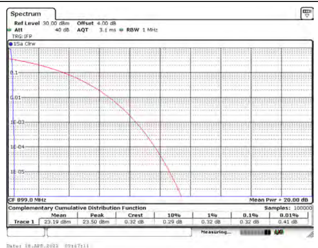
3.75 kHz / QPSK / CH21627 / 1RB0
