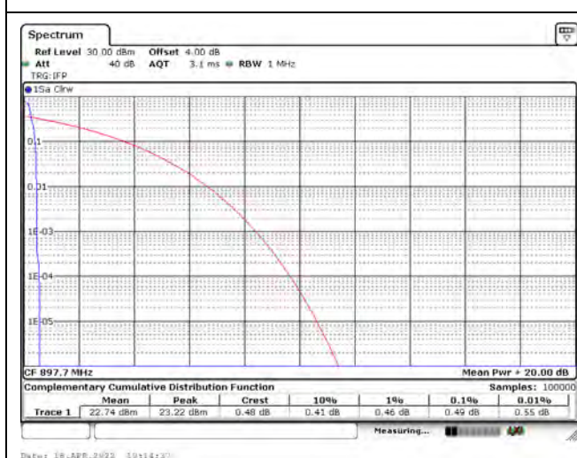
15 kHz / BPSK / CH21627 / 1RB0
