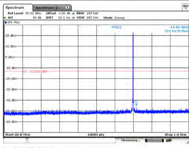
15 kHz / QPSK / CH134180 / 1RB11 / Below 1 GHz
