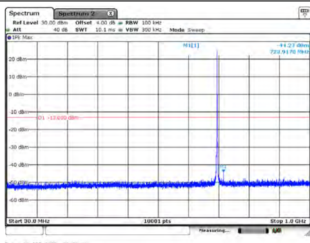
10 MHz / QPSK / CH134132 / 1RB5 / Below 1 GHz
