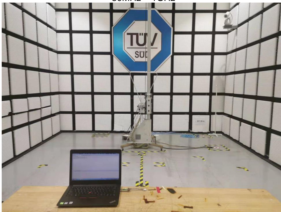
30MHz ~ 1GHz
