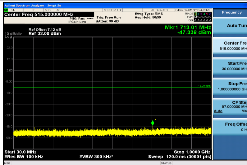
Band4-1.4MHz-QPSK-20393-1RB#0-30~1000MHz
