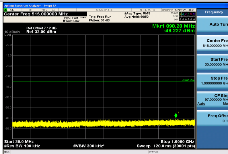
Band2-20MHz-QPSK-18700-1RB#0-30~1000MHz
