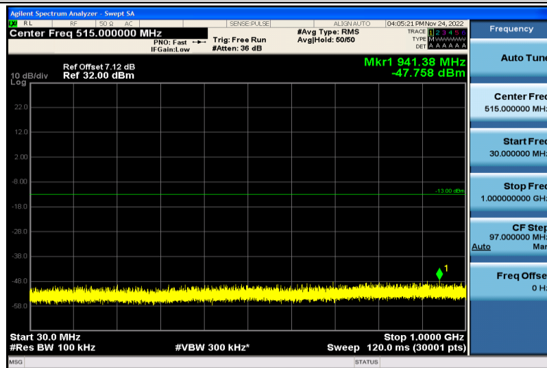
Band2-20MHz-16QAM-18700-1RB#0-30~1000MHz
