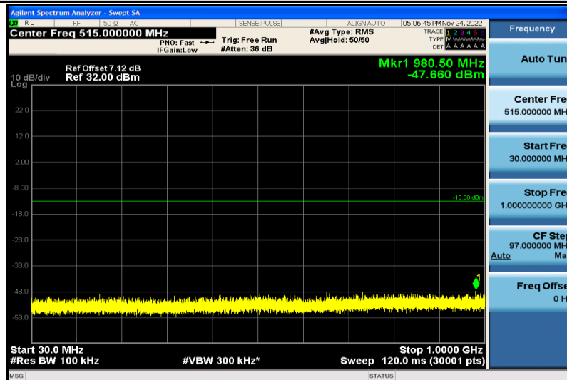
Band4-3MHz-QPSK-20385-1RB#0-30~1000MHz
