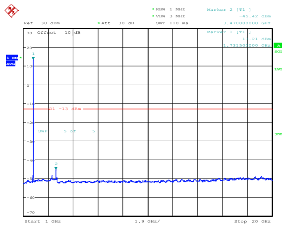
Band4-20MHz-QPSK-20300-1RB#0-Range4:1000~20000MHz
