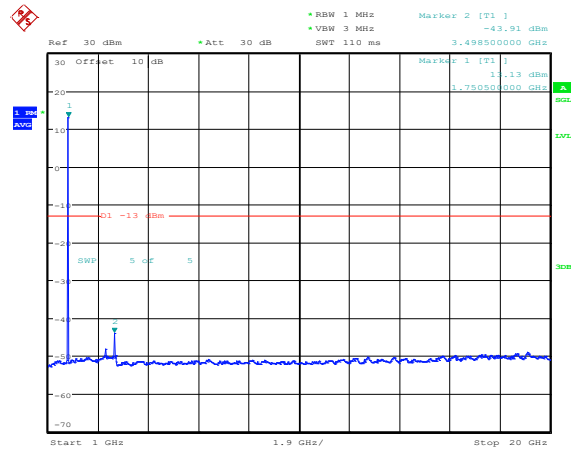
Band4-5MHz-QPSK-20375-1RB#0-Range4:1000~20000MHz
