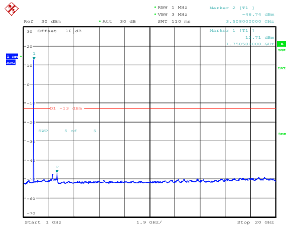
Band4-1.4MHz-QPSK-20393-1RB#0-Range4:1000~20000MHz
