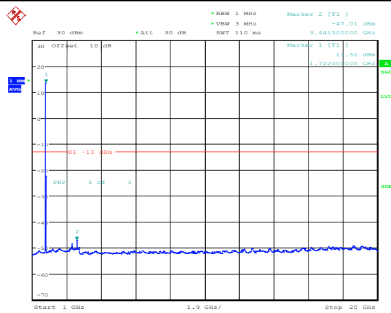
Band4-20MHz-QPSK-20175-1RB#0-Range4:1000~20000MHz
