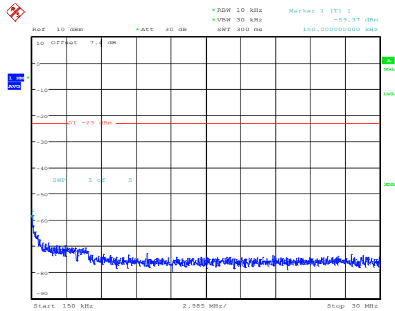
Band4-3MHz-QPSK-20175-1RB#0-Range2:0.15~30MHz
