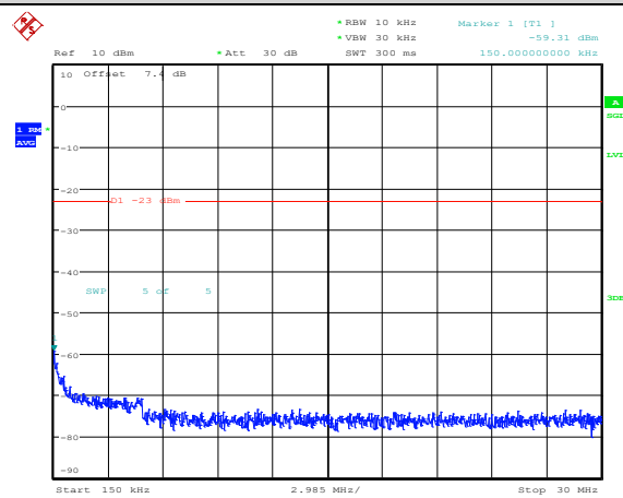
Band4-1.4MHz-QPSK-19957-1RB#0-Range2:0.15~30MHz
