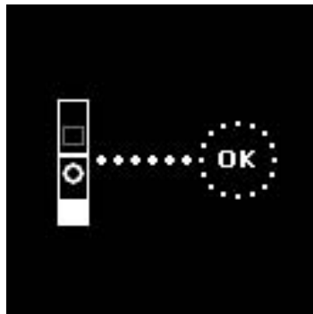
Verbindung erfolgreich
