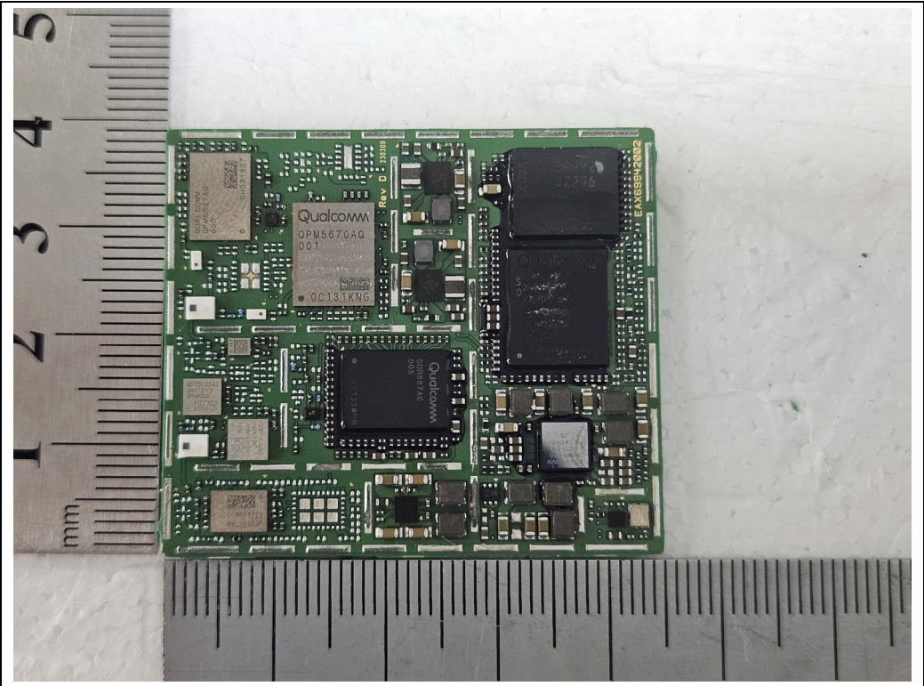
<LTE Module>
