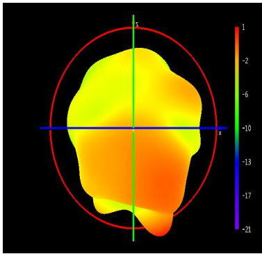
Theta=90 freq=2400MHz
