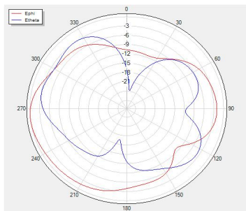
Theta=90 freq=2400MHz
