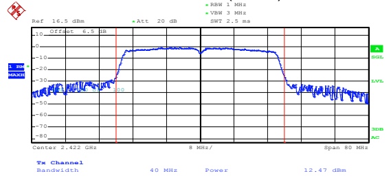
802.11n(HT40)
