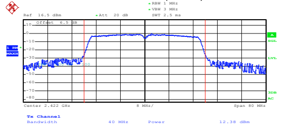
802.11n(HT40)
