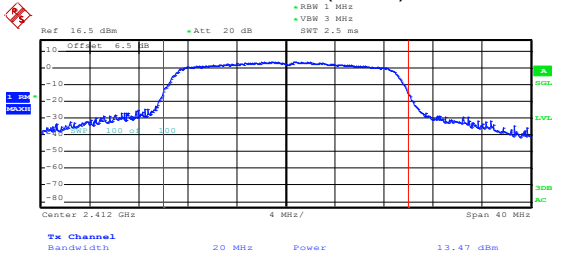
802.11n(HT20)
