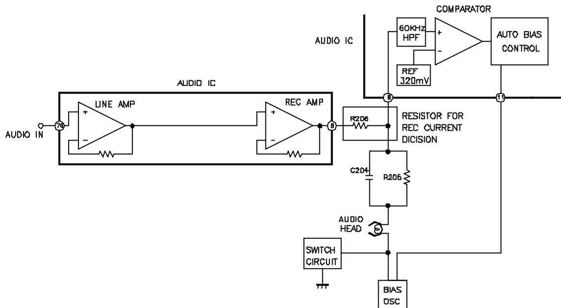
Fig. 4-2 REC mode
