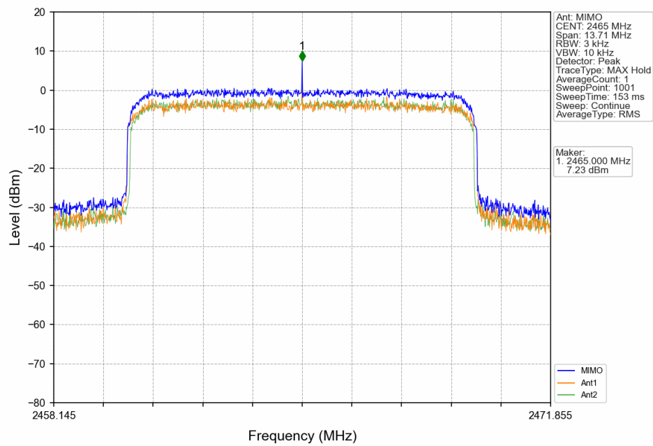
Slot10_HCH_2465MHz_MIMO_NTNV
