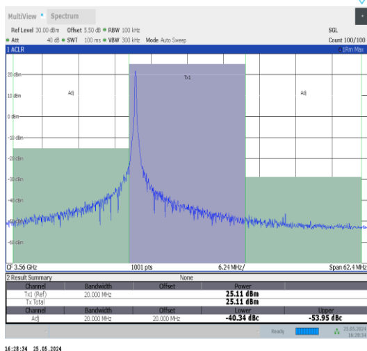
Band48-20MHz-QPSK-55340-1RB#0-PASS
