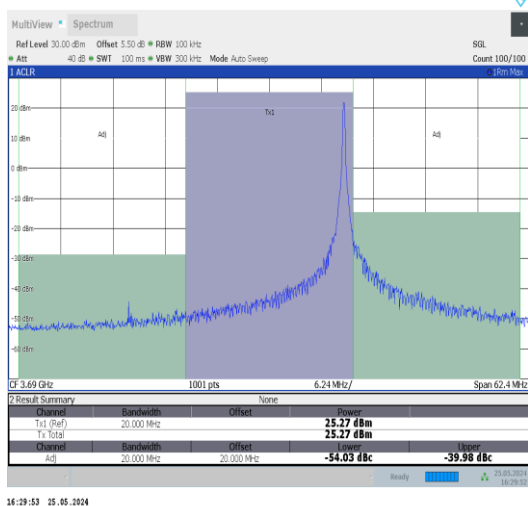
Band48-20MHz-QPSK-56640-1RB#99-PASS
