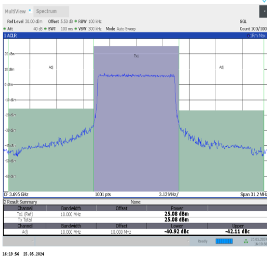
Band48-10MHz-QPSK-56690-50RB#0-PASS
