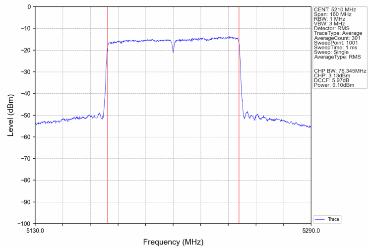
802.11ac(VHT80)_MCH_5210MHz_Ant2_NTNV
