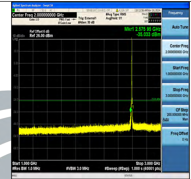
Band41 5MHz QPSK 40590 1RB#0 1000~3000 1000~3000
