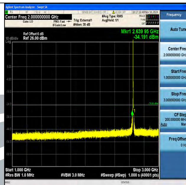
Band41 5MHz QPSK 41215 1RB#0 1000~3000 1000~3000
