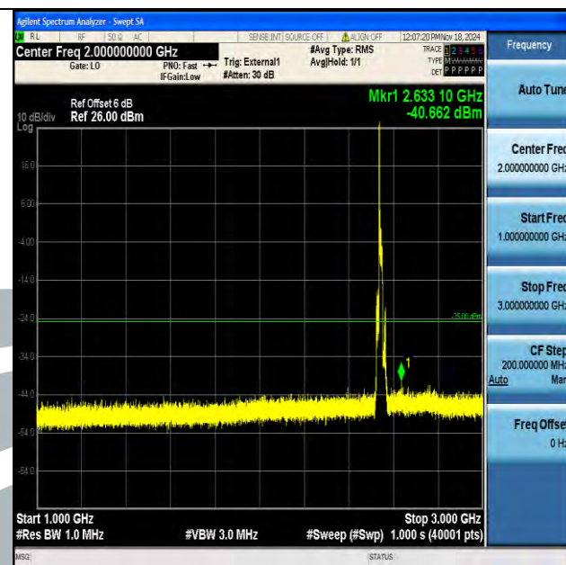
Band41 15MHz QPSK 40115 1RB#0 1000~3000 1000~3000
