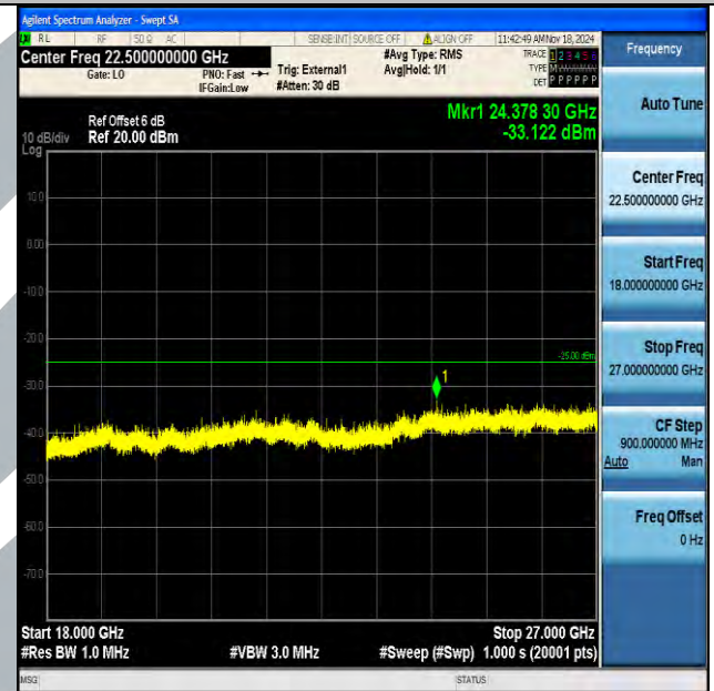
Band41_10MHz_16QAM_41190_1RB#0_18000~27000_18000~27000
