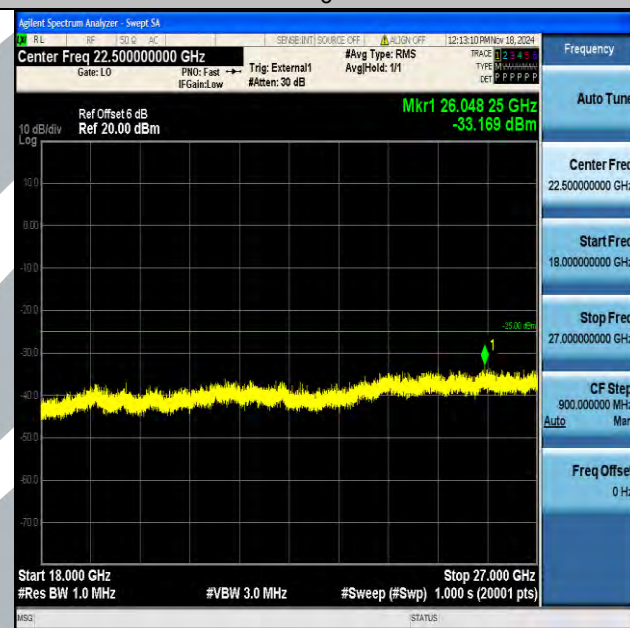
Band41_15MHz_16QAM_40590_1RB#0_18000~27000_18000~27000
