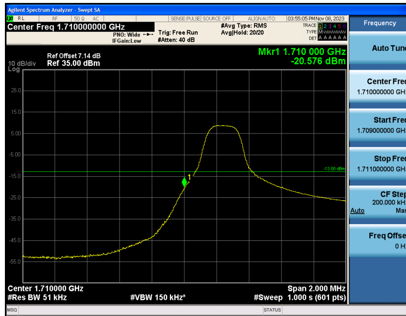
Band4-3MHz-QPSK-19965-1RB#14
