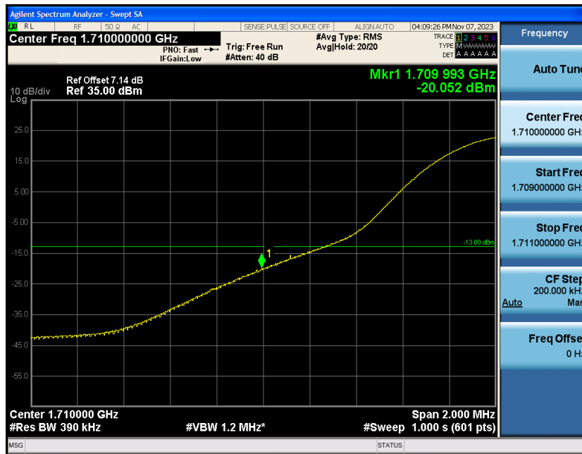
Band4-20MHz-QPSK-20050-1RB#99
