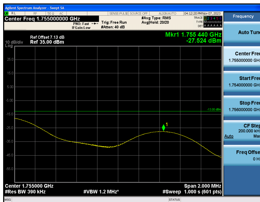
Band4-20MHz-QPSK-20300-1RB#99
