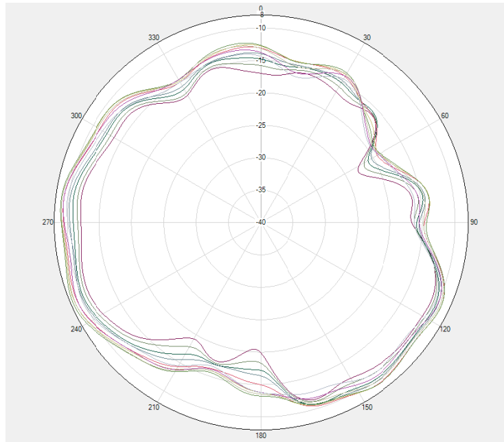
GSM850 / WCDMA B5 / LTE B5/B20 \Phi=90\text{deg}
