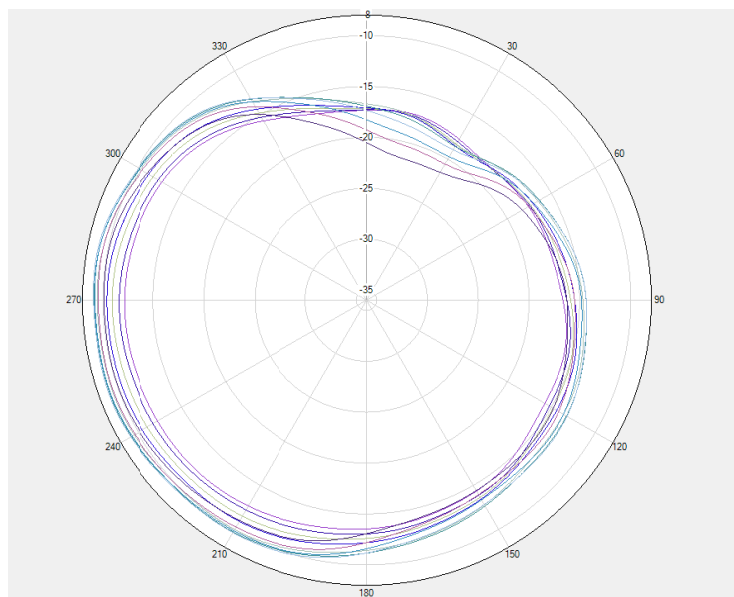
GSM850 / WCDMA B5 / LTE B5/B20 \Theta=90\text{deg}
