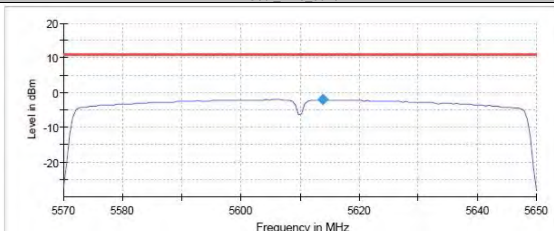
11AC80 Ant5 5610
