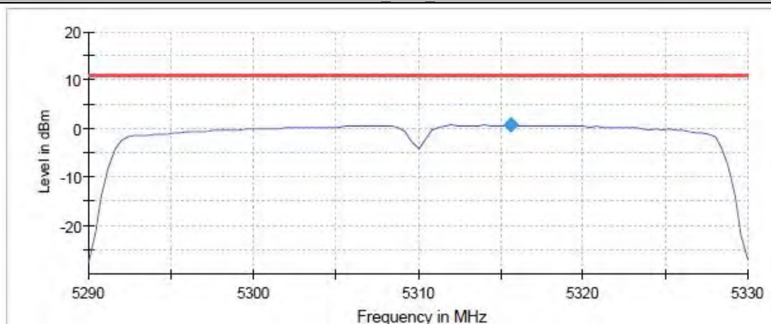
11AC40 Ant6 5310
