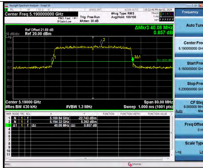
11AX40MIMO_Ant6_5190
