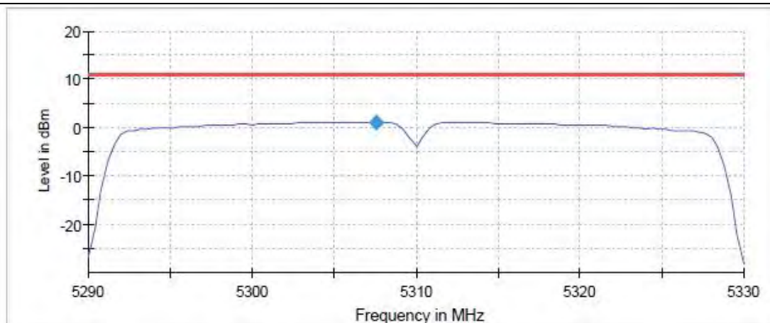
11AC40 Ant6 5310
