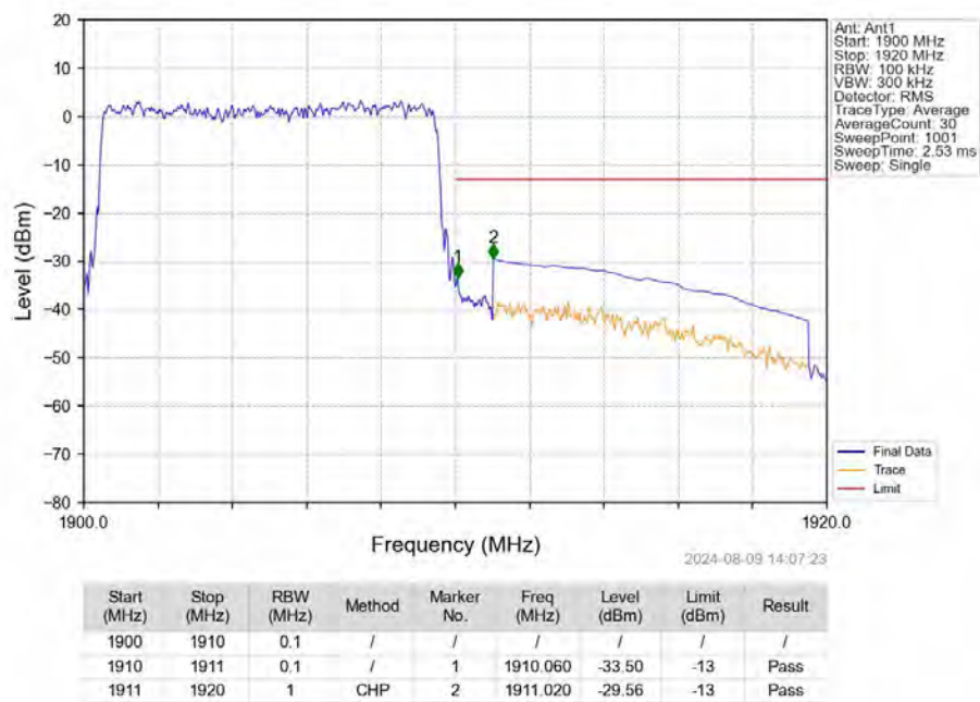
Band2_10MHz_16QAM_HCH_1905MHz_RB_50_0_NTNV
