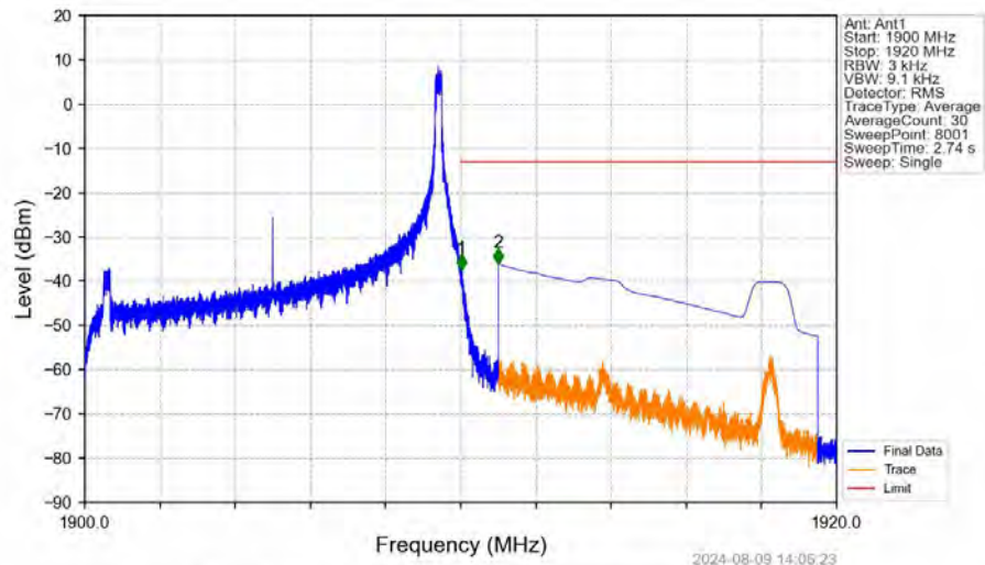
Band2_10MHz_QPSK_HCH_1905MHz_RB_1_49_NTNV
