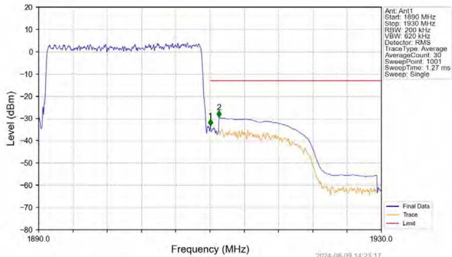
Band2_20MHz_QPSK_HCH_1900MHz_RB_100_0_NTNV
