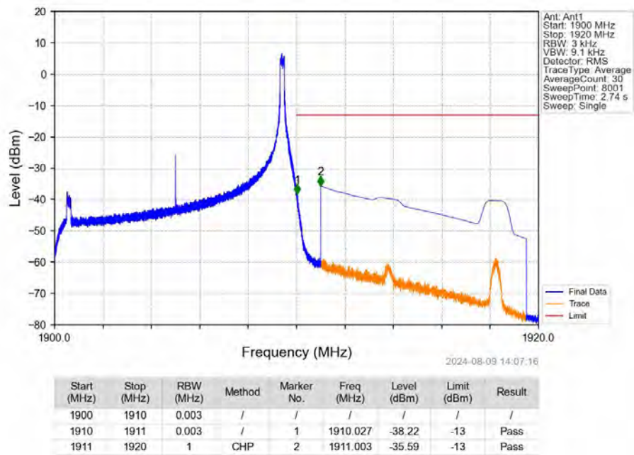
Band2_10MHz_16QAM_HCH_1905MHz_RB_50_0_NTNV
