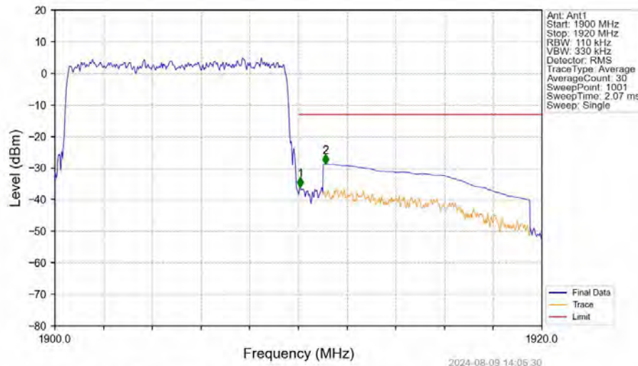
Band2_10MHz_QPSK_HCH_1905MHz_RB_50_0_NTNV
