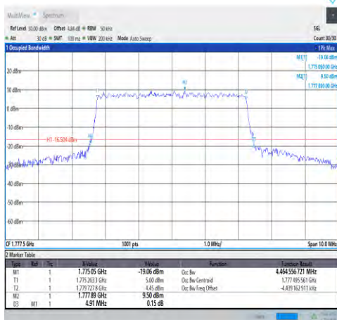
1-N66-PC3-15-5-H-7-CP-16QAM-Outer_Full-25@0-Ant1-4.465-4.910-≤5-PASS
