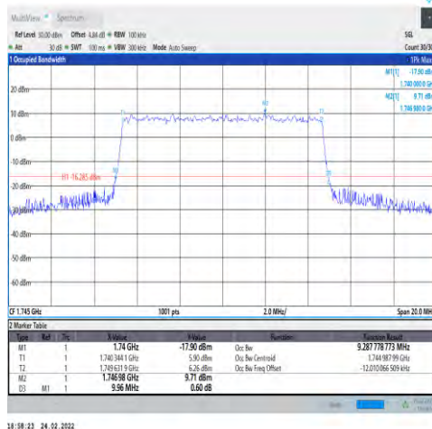
1-N66-PC3-15-10-M-7-CP-16QAM-Outer_Ful I-52@0-Ant1-9.288-9.960-≤10-PASS
