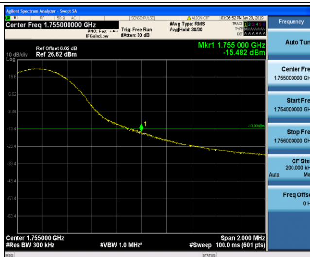
Band4 15MHz QPSK 20325 1RB#74
