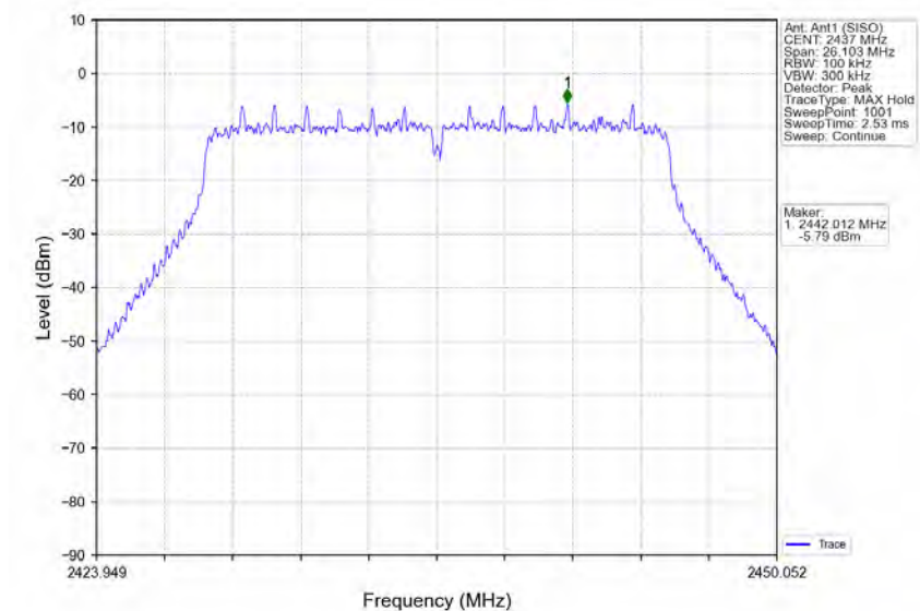
802.11n(HT20)_MCH_2437MHz_Ant1 (SISO)_NTNV
