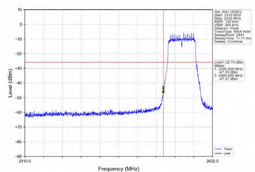
802.11n(HT20)_LCH_2412MHz_Ant1 (SISO)_NTNV
