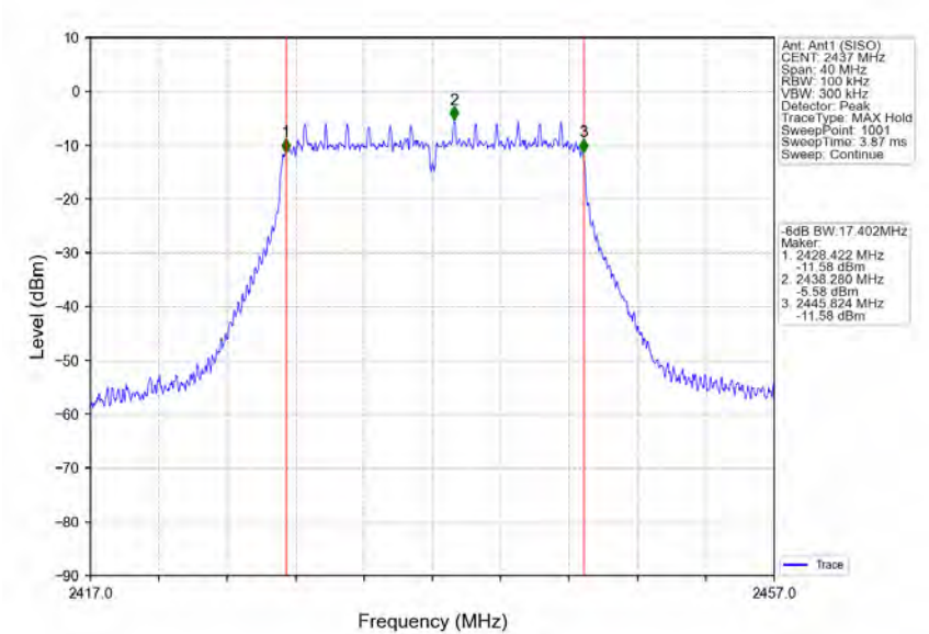
802.11n(HT20)_MCH_2437MHz_Ant1 (SISO)_NTNV
