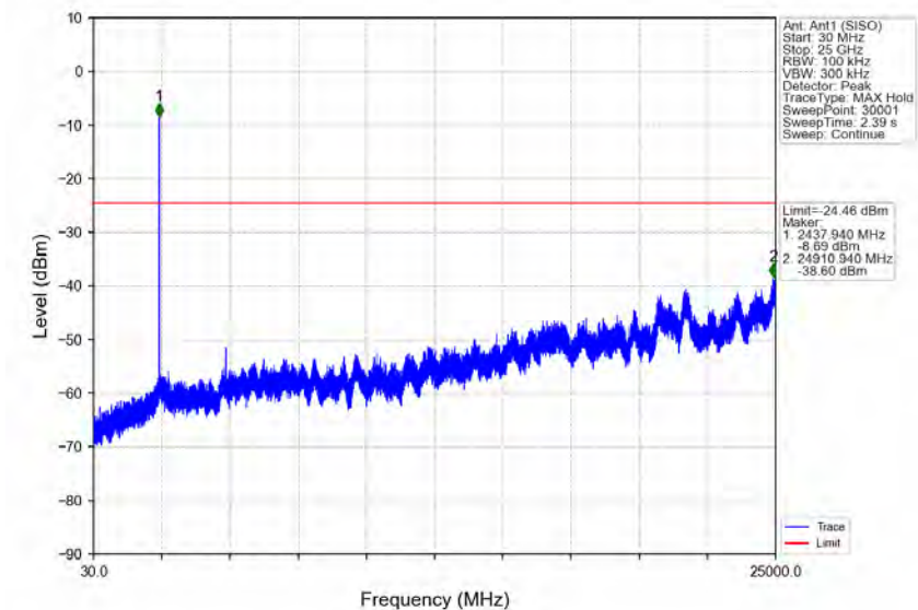
802.11g_MCH_2437MHz_Ant1 (SISO)_NTNV
